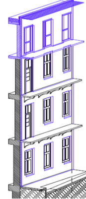
UTÓLAGOS HŐSZIGETELÉS A BELSŐ HOMLOKZATOKON, SZINTÉRÁPÍTÉS AZ UDVARI OLDALON
