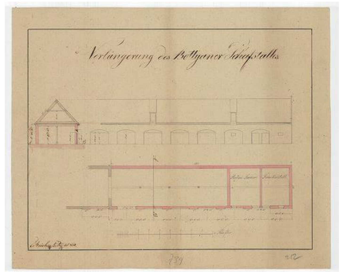
No 739 A kibővítendő bottyányi (Somogy m.) juhakol
