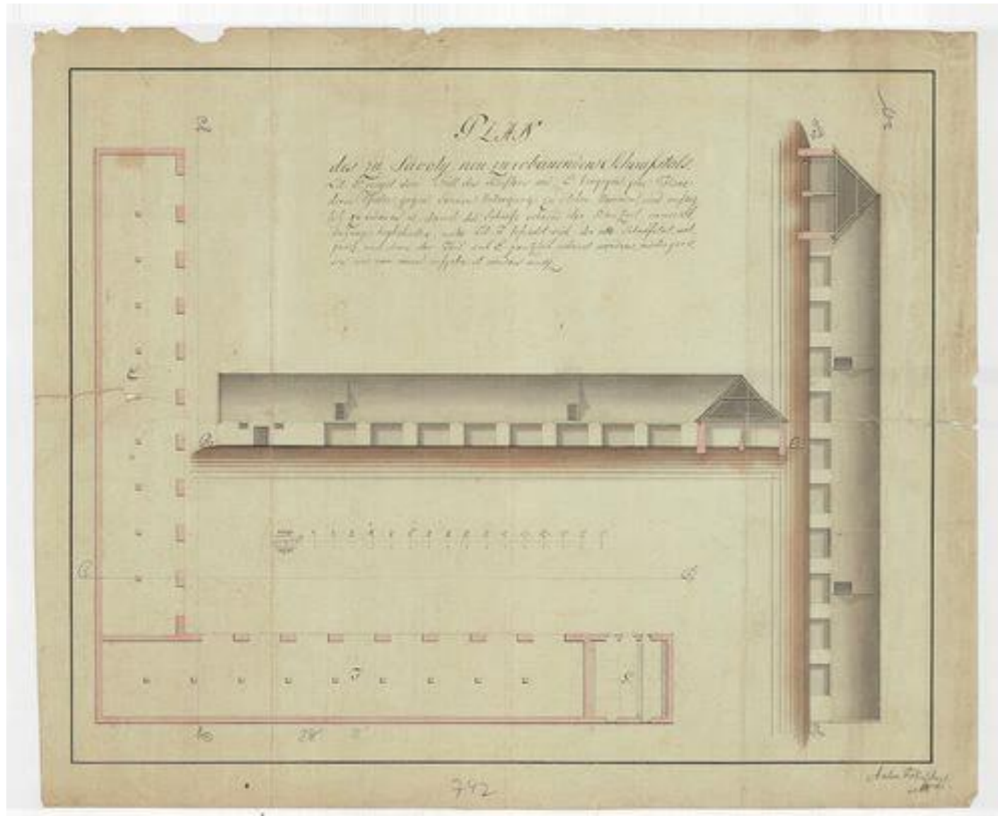
No 742 A tervezett sávolyi (Somogy m.) juhakol
