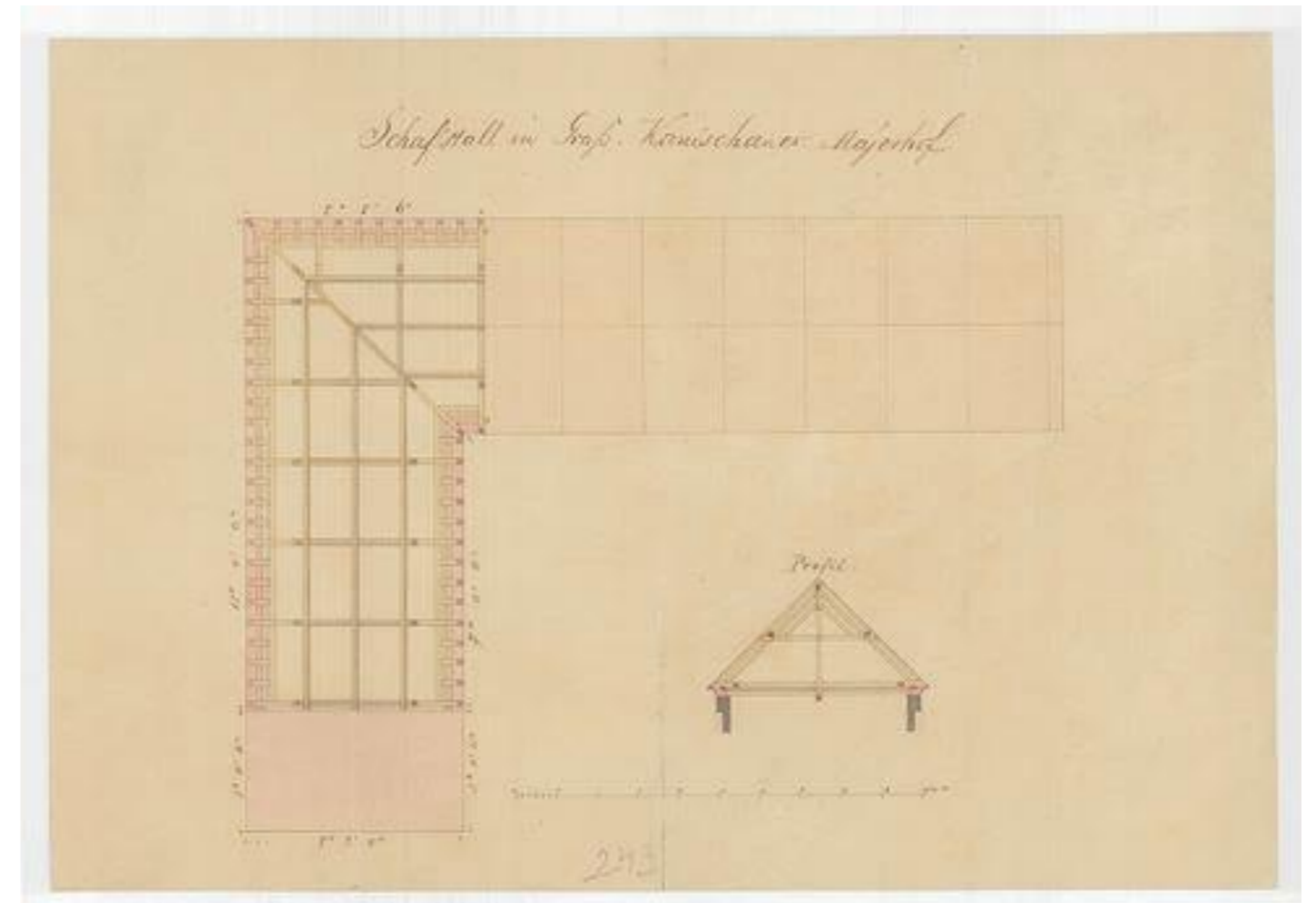
No. 243. A nagykanizsai juhakol és a tetőzet
