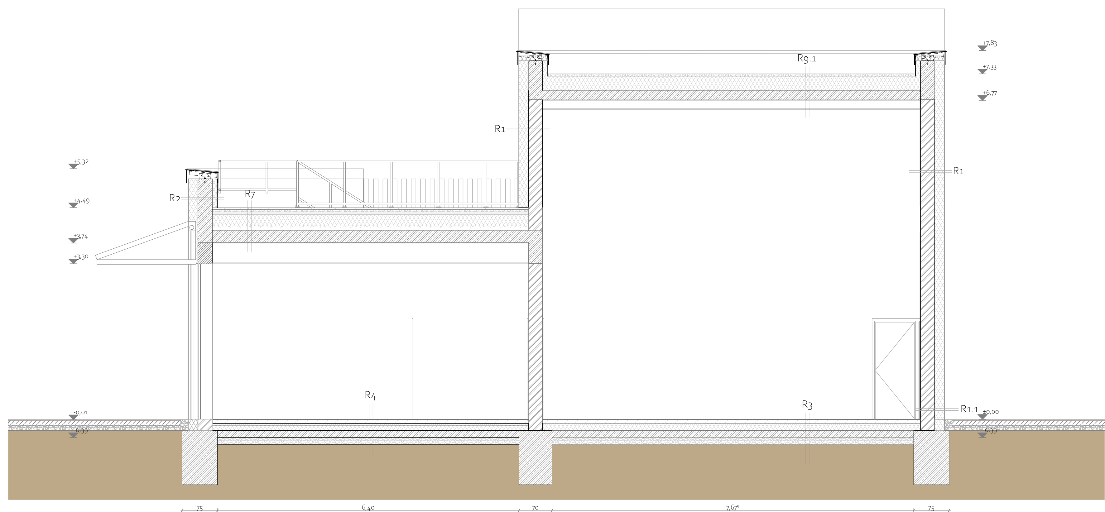
C-C metszet M = 1:100
