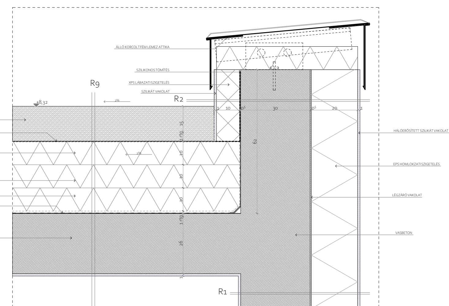
Attika csomópont M = 1:10
