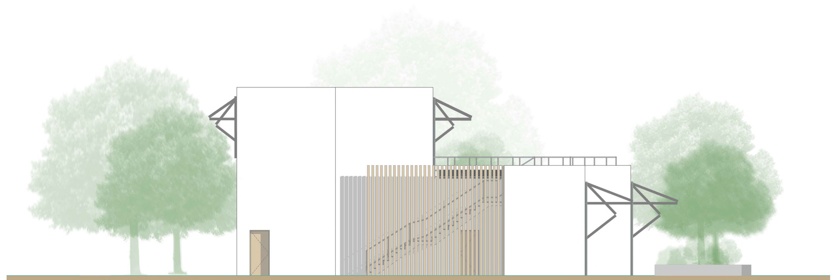
Nyugati homlokzat M = 1:100
