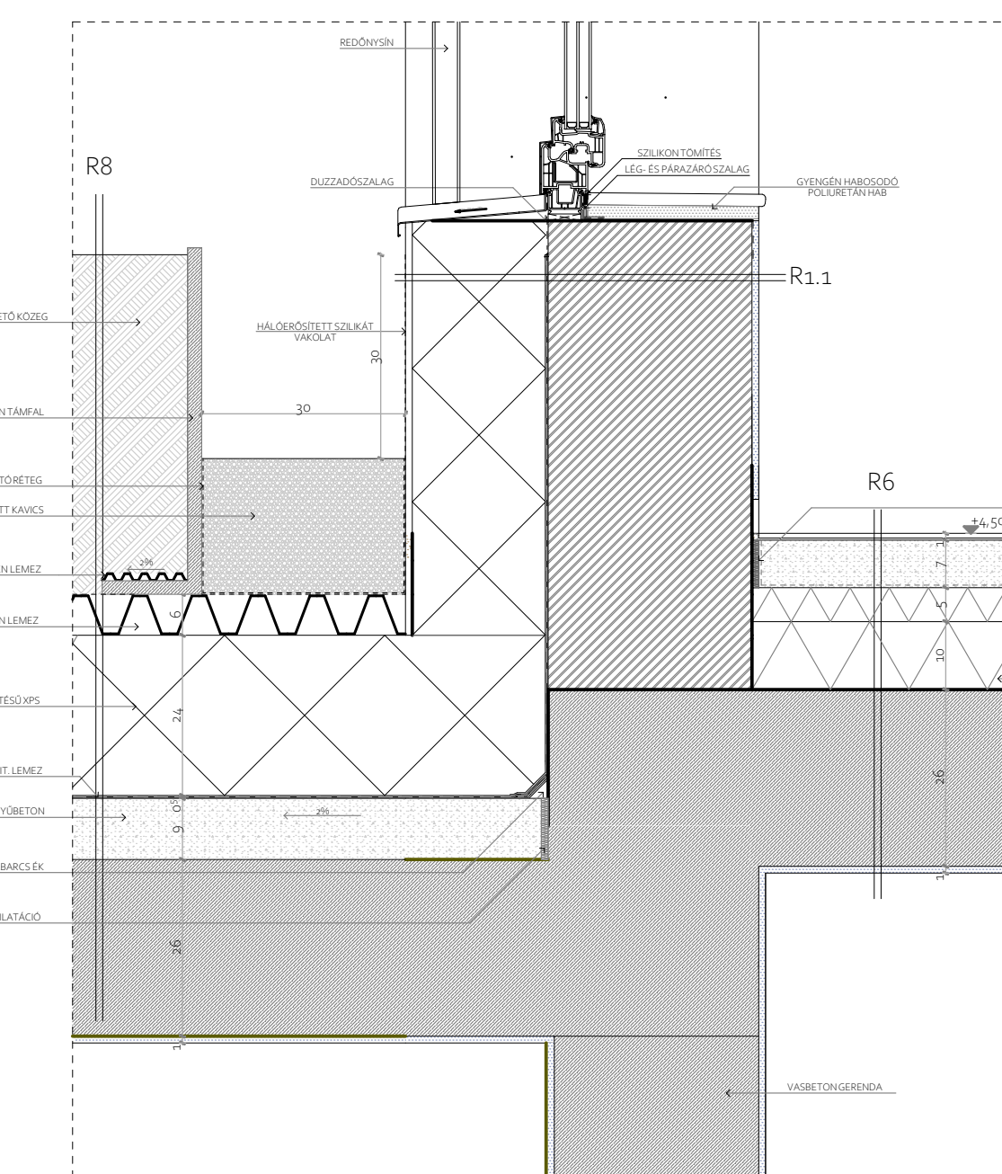
Ablak alsó csomópont M = 1:10
