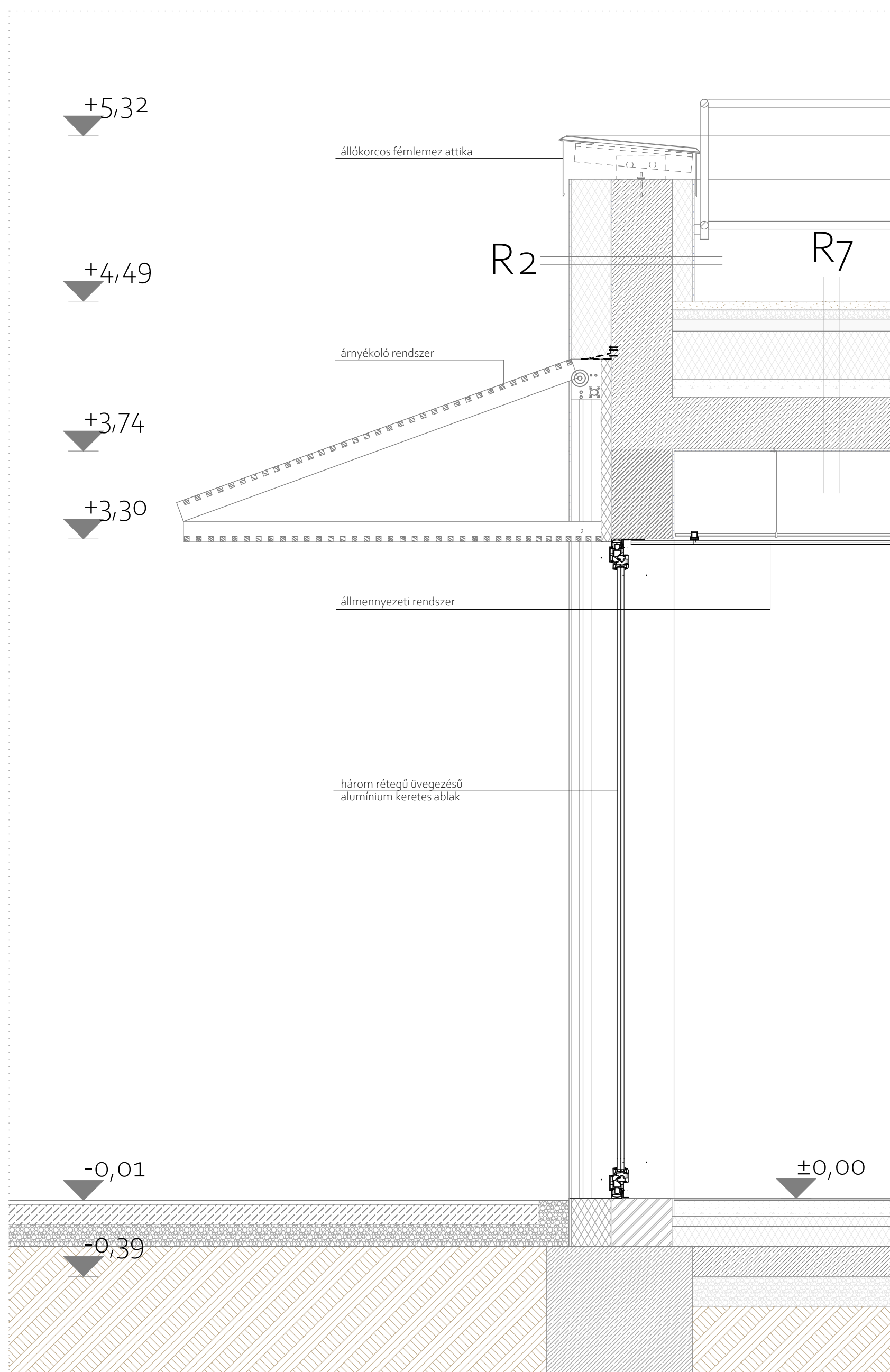
Metszet részlet M = 1:20
