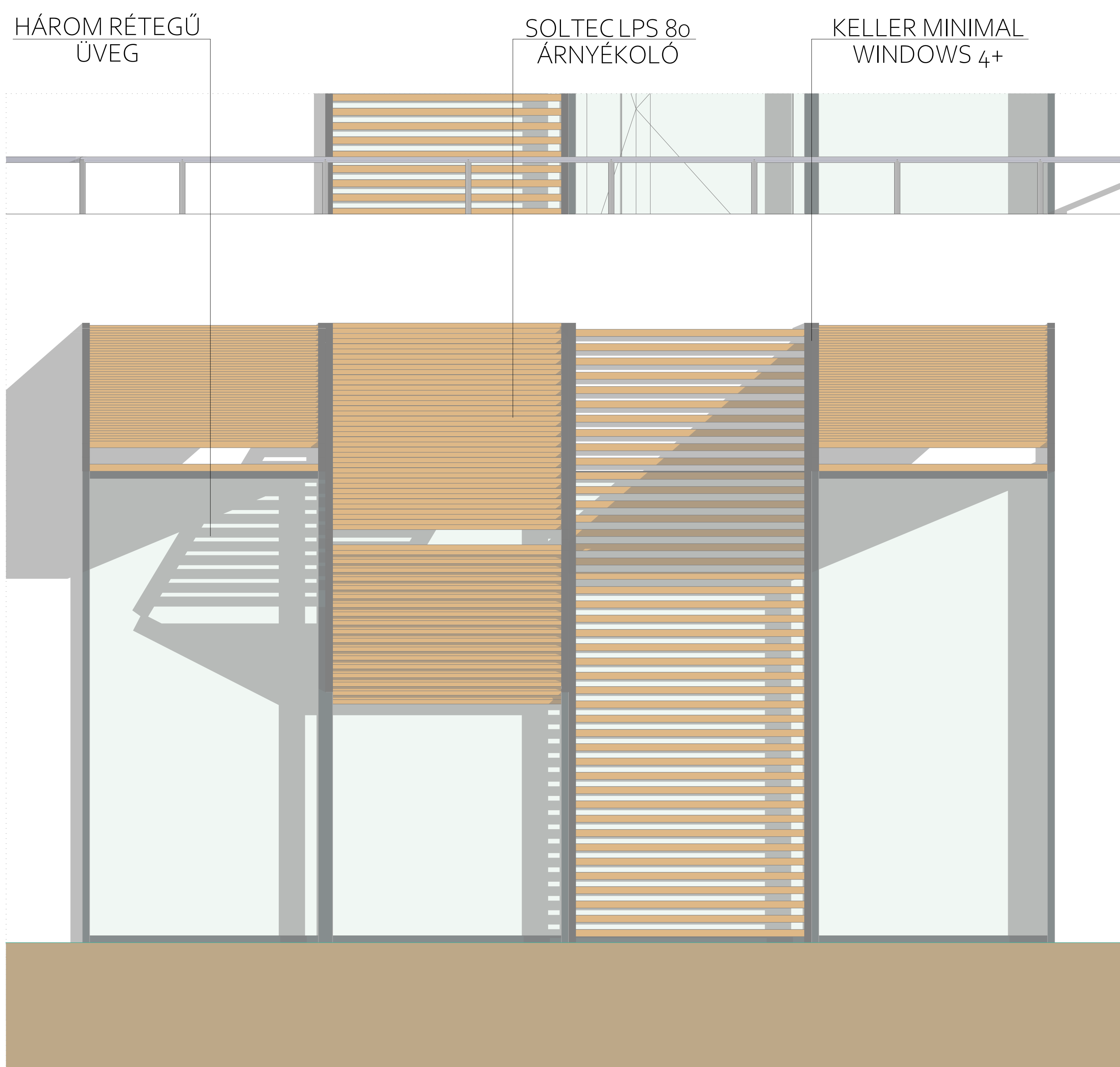
Homlokzat részlet M = 1:20
