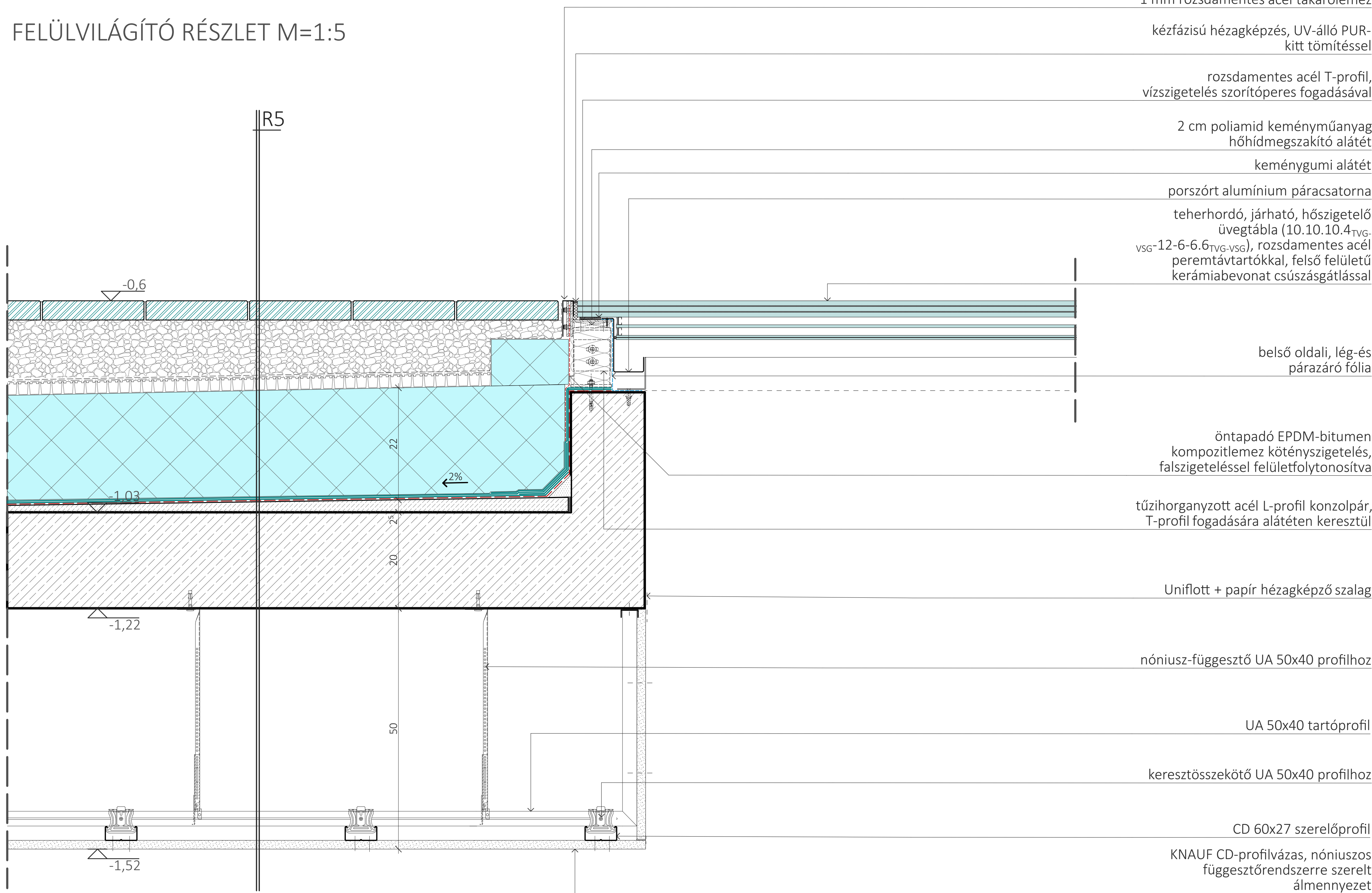
HOMLOKZATI RÉSZLETEK M=1:5
