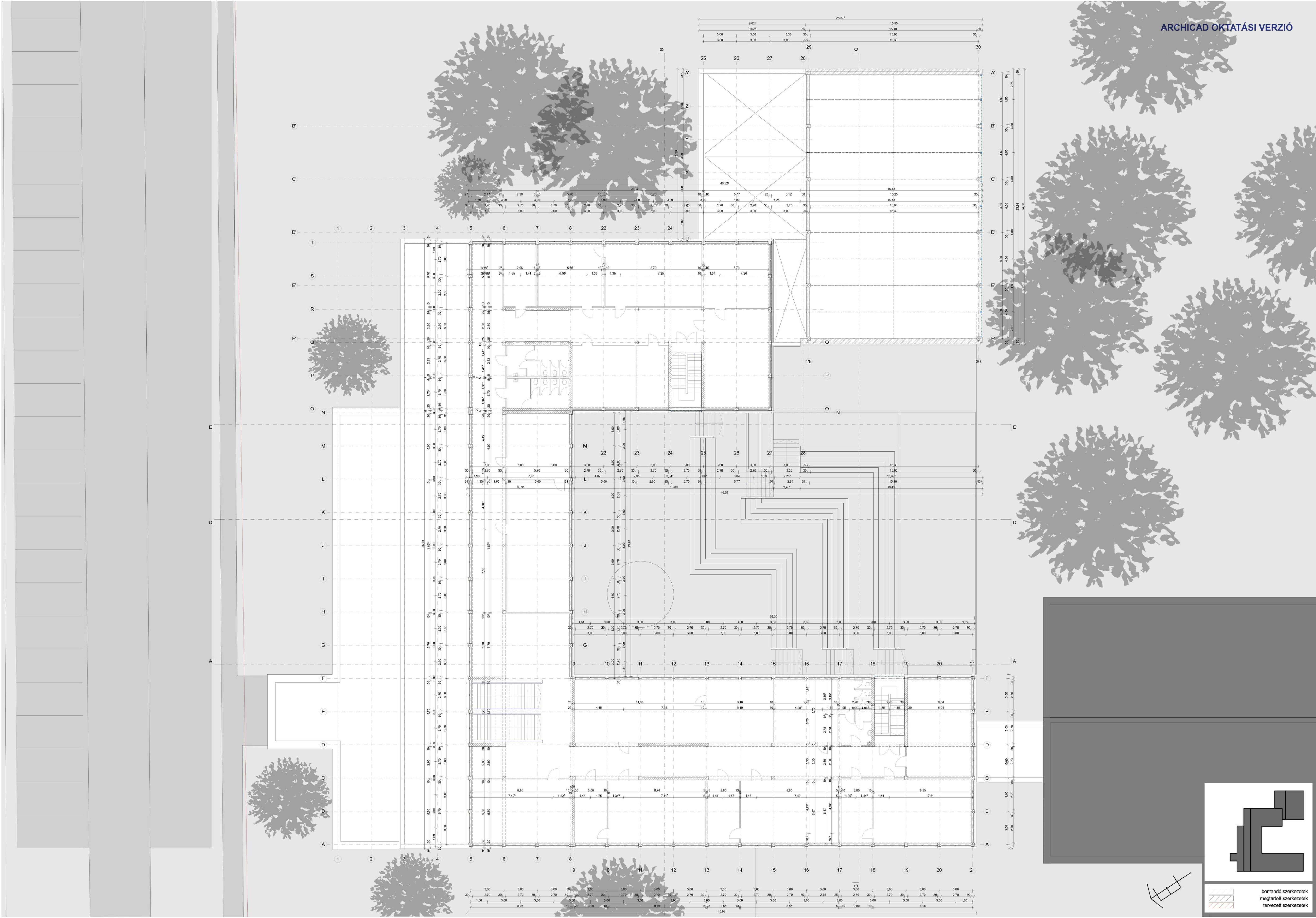
II. EMELETI ALAPRAJZ / MEGLÉVŐ ÁLLAPOT / M = 1:150
