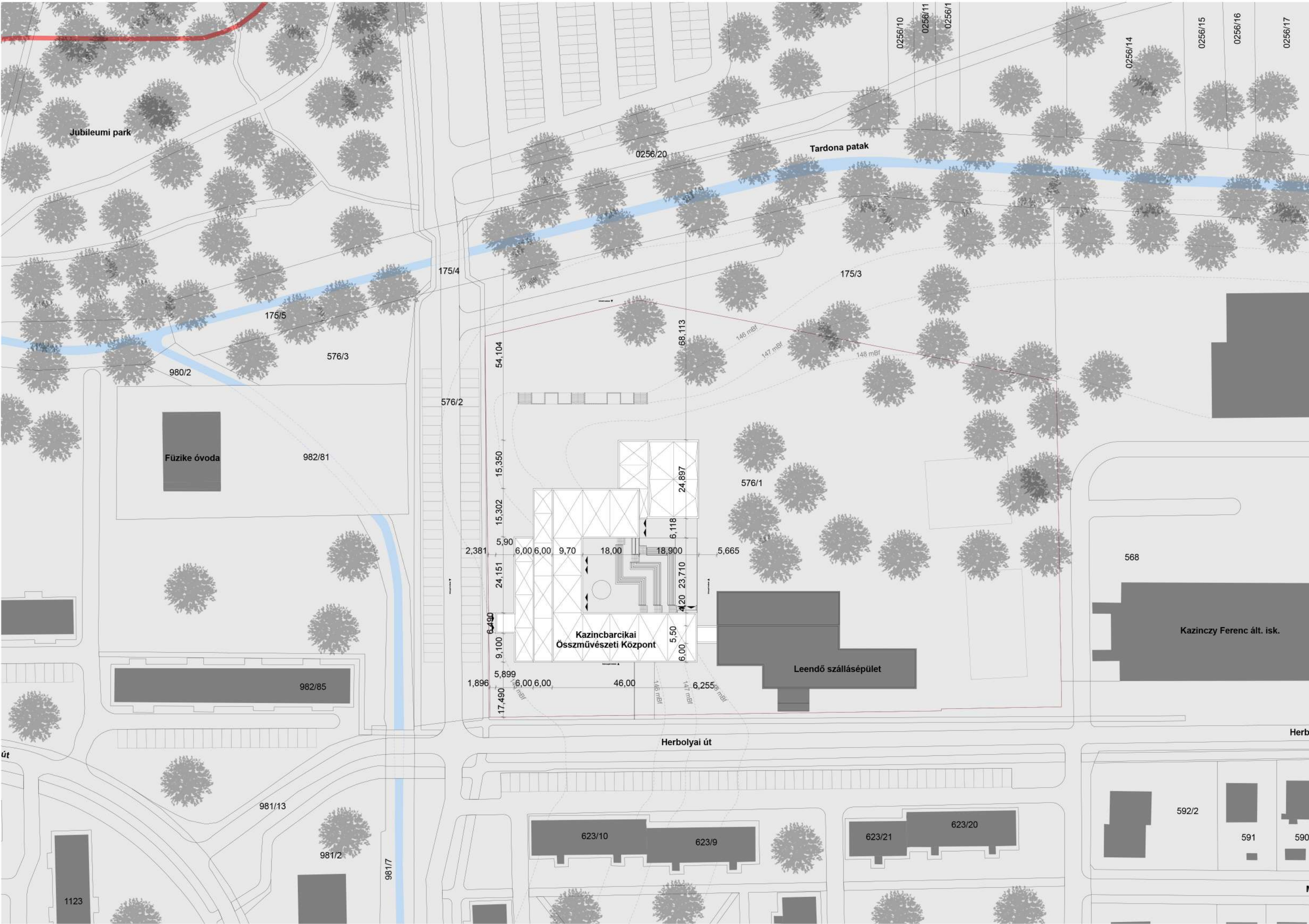
MEGLÉVŐ HELYSZÍNRAJZ / M = 1:1000
