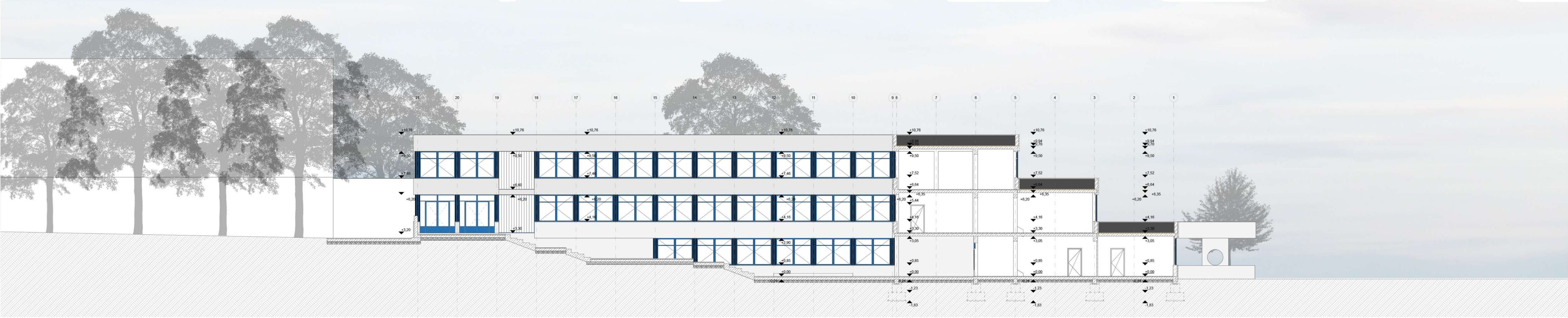
D – D METSZET / MEGLÉVŐ ÁLLAPOT / M = 1:150
