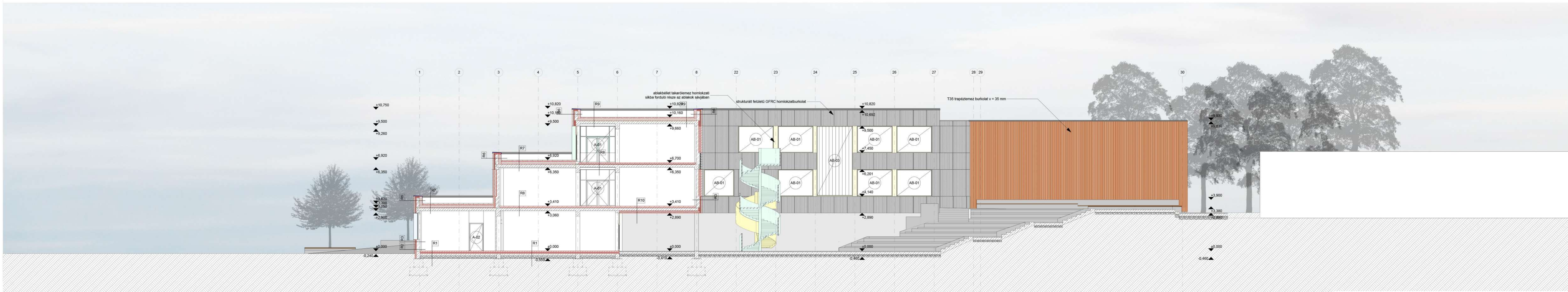
A – A METSZET / TERVEZETT ÁLLAPOT / M = 1:150
