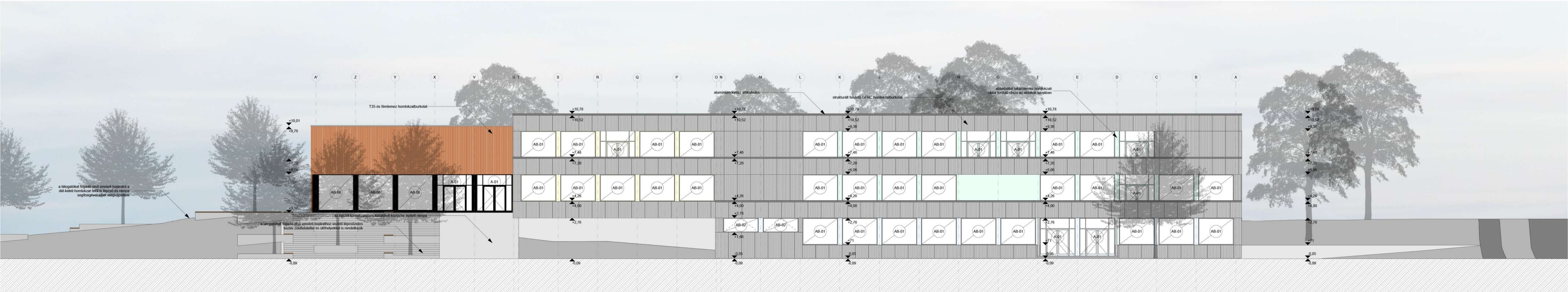
ÉSZAK-KELETI HOMLOKZAT / TERVEZETT ÁLLAPOT / M = 1:150
