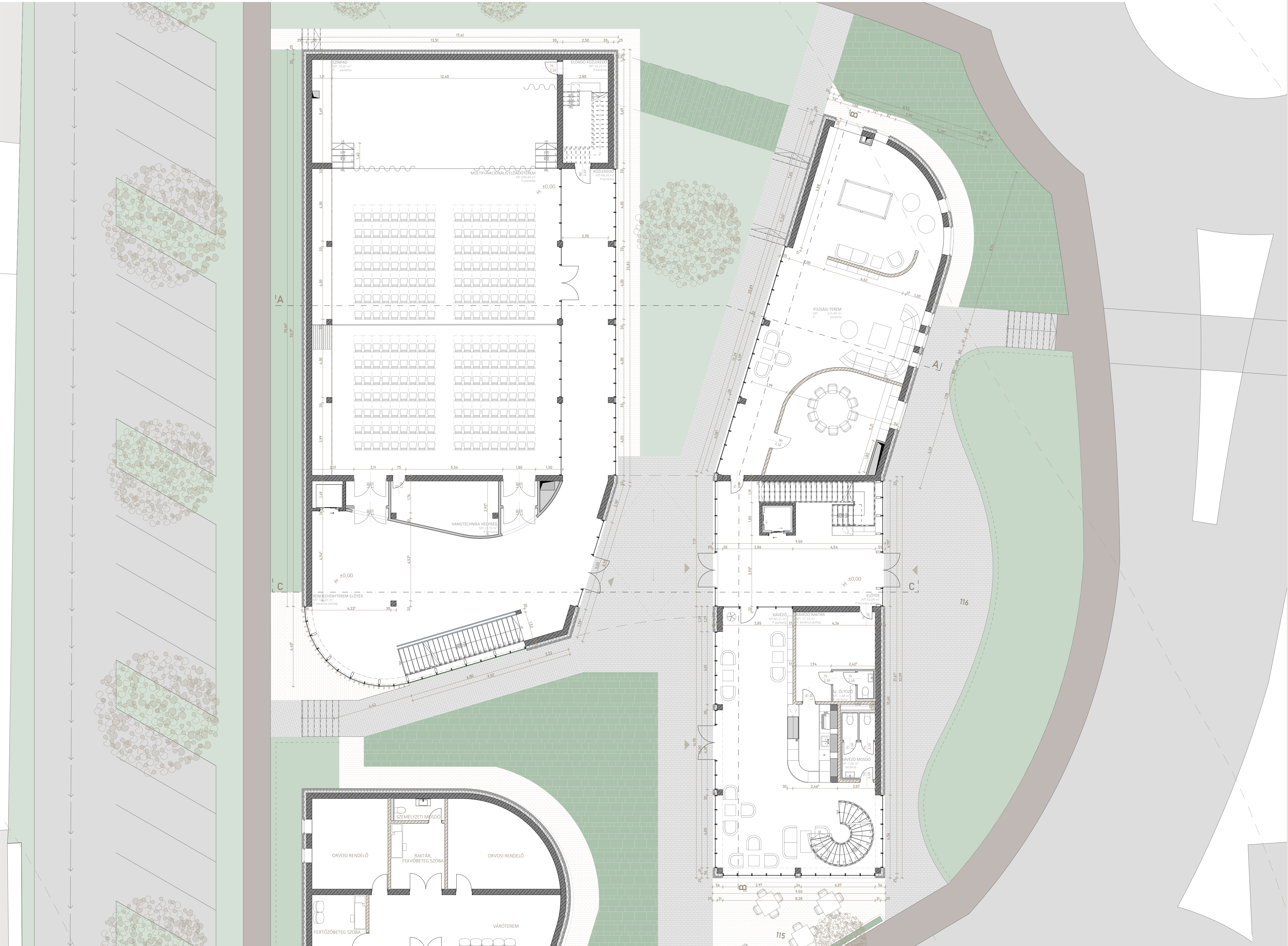
FÖLDSZINTI ALAPRAJZ 1:100
