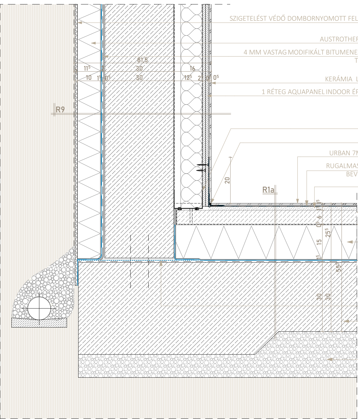
PINCESZINT ALAPOZÁS 1:10
