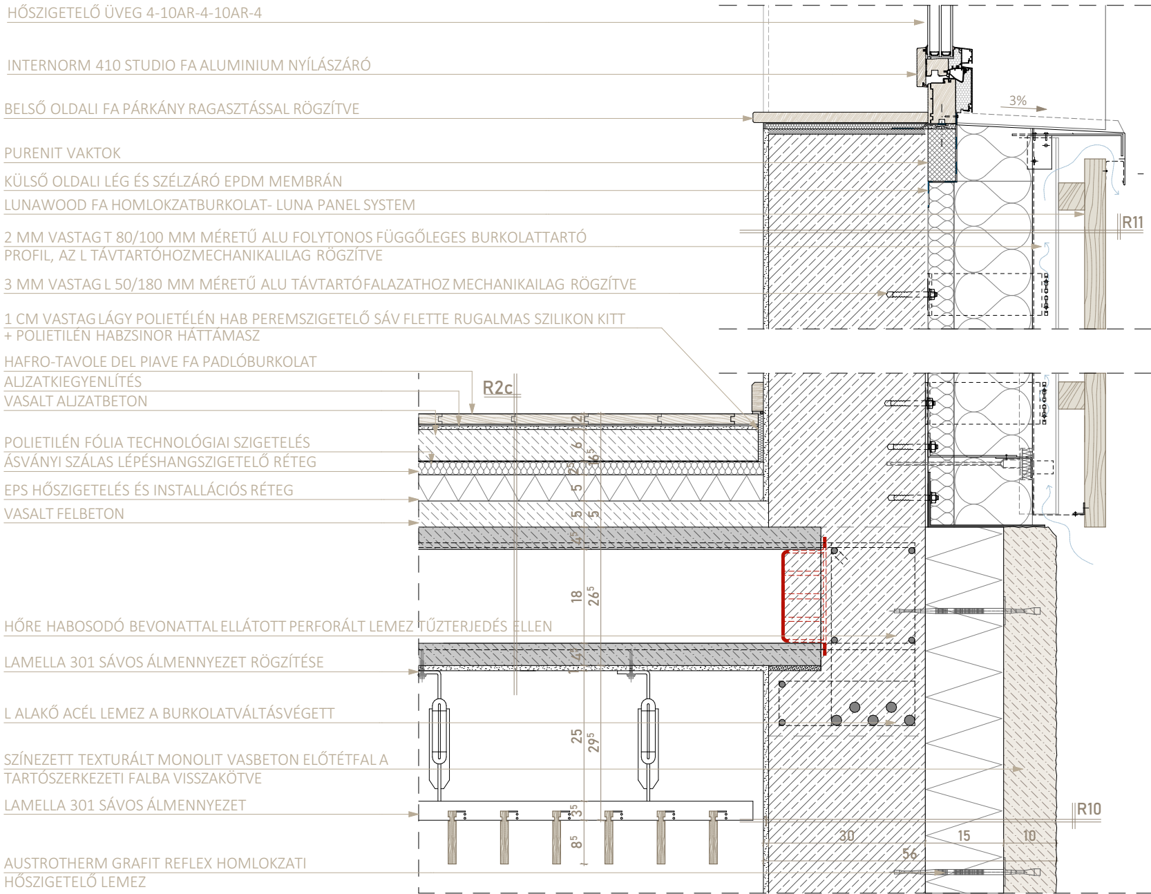
BURKOLATVÁLTÁS ABLAK BEÉPÍTÉS 1:10
