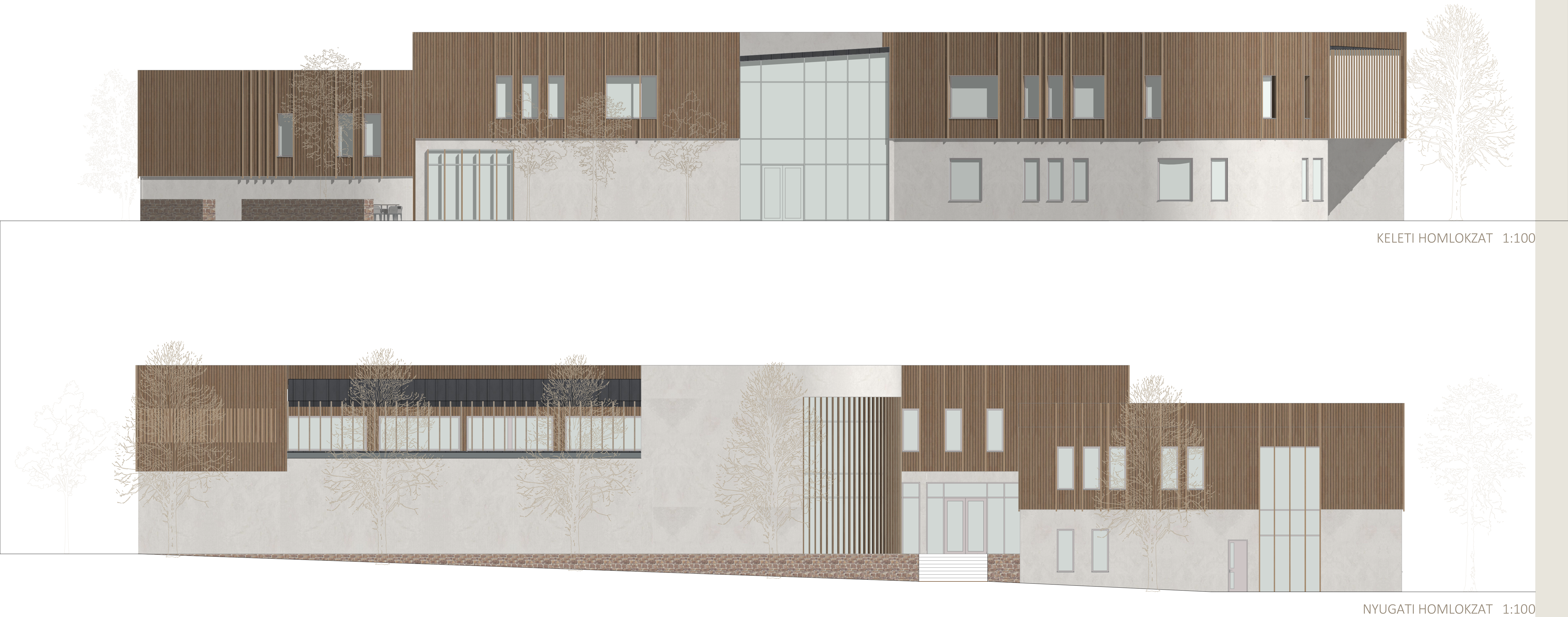
NYUGATI HOMLOKZAT 1:100
