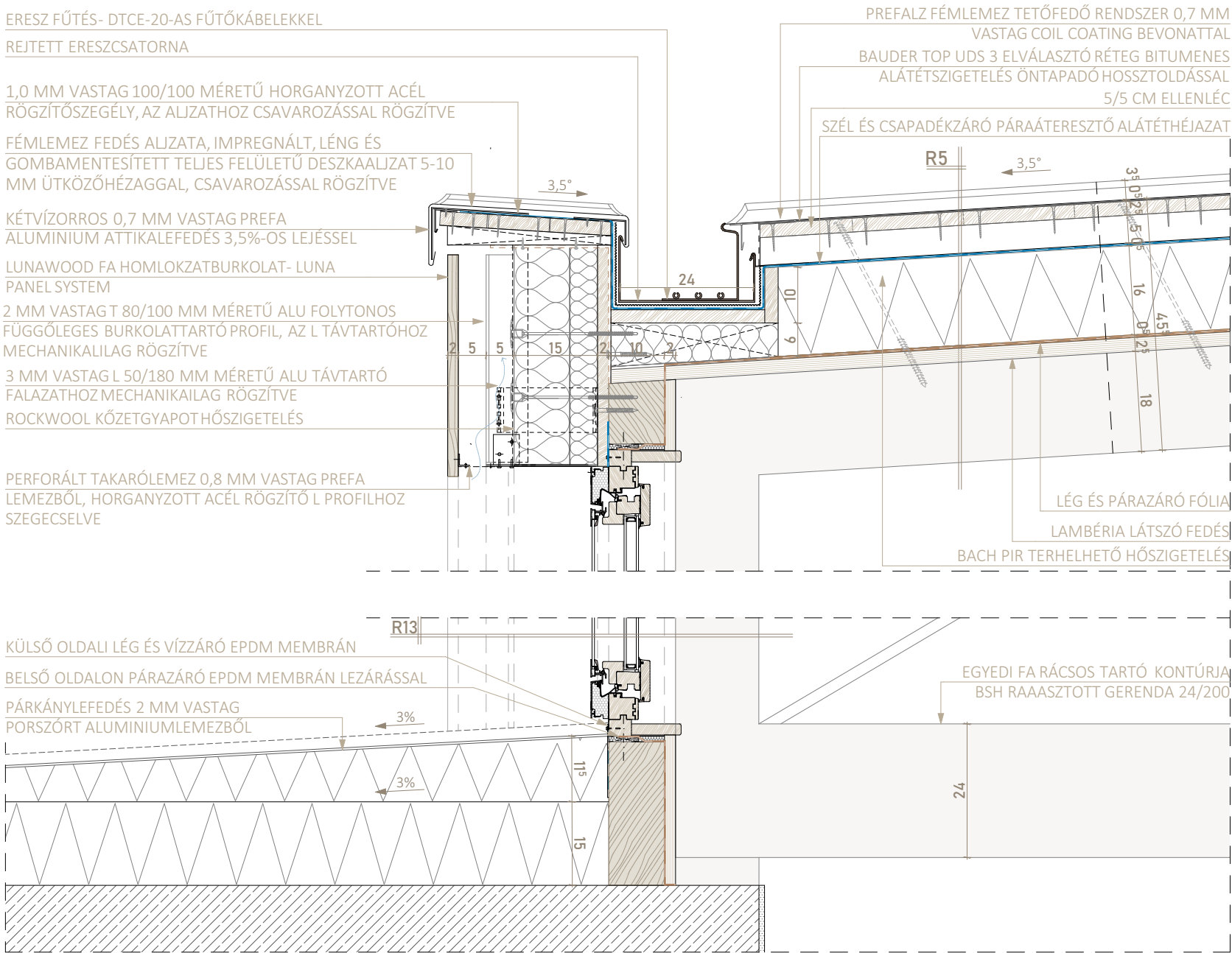
RENDEZVÉNYTEREM REJTETT ERESZ 1:10
