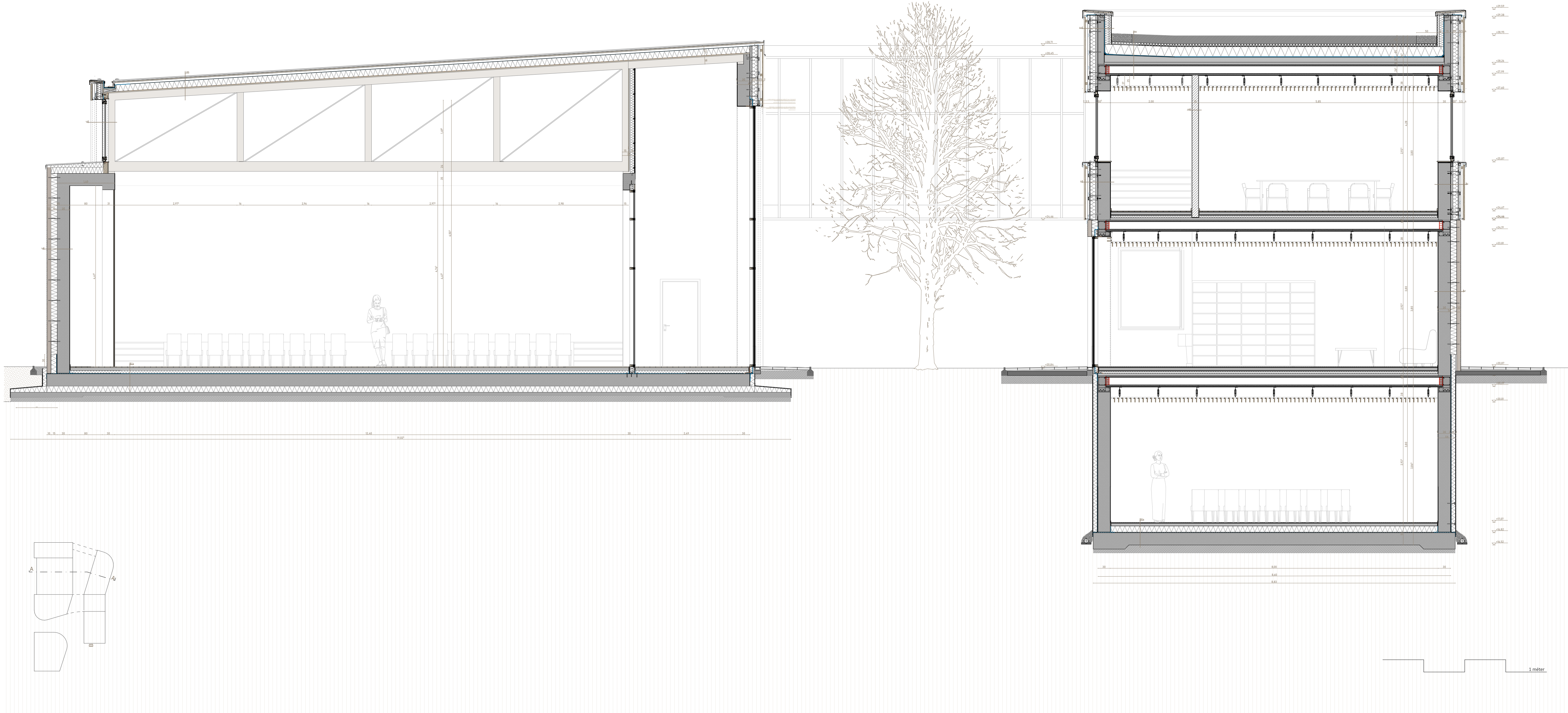
A-A METSZET 1:50
