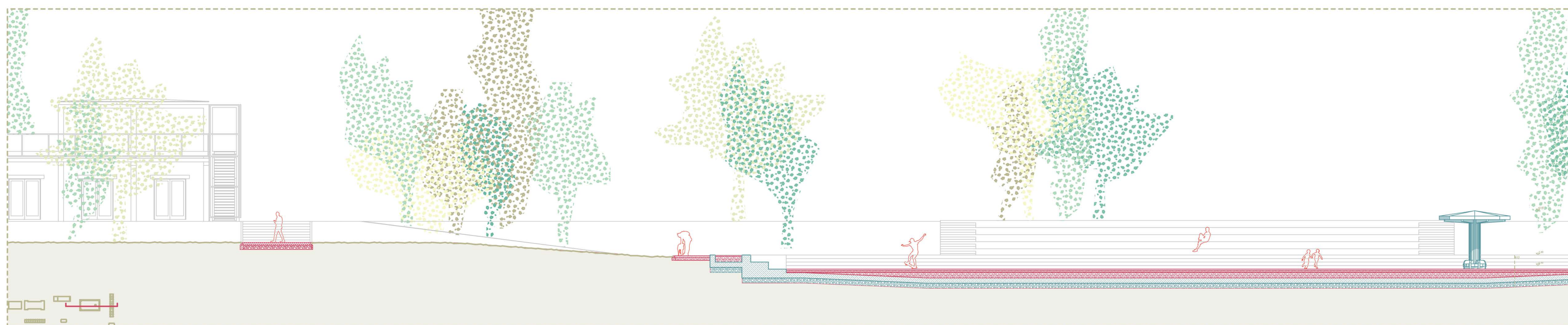
Gömbs medence metszet 1:100
