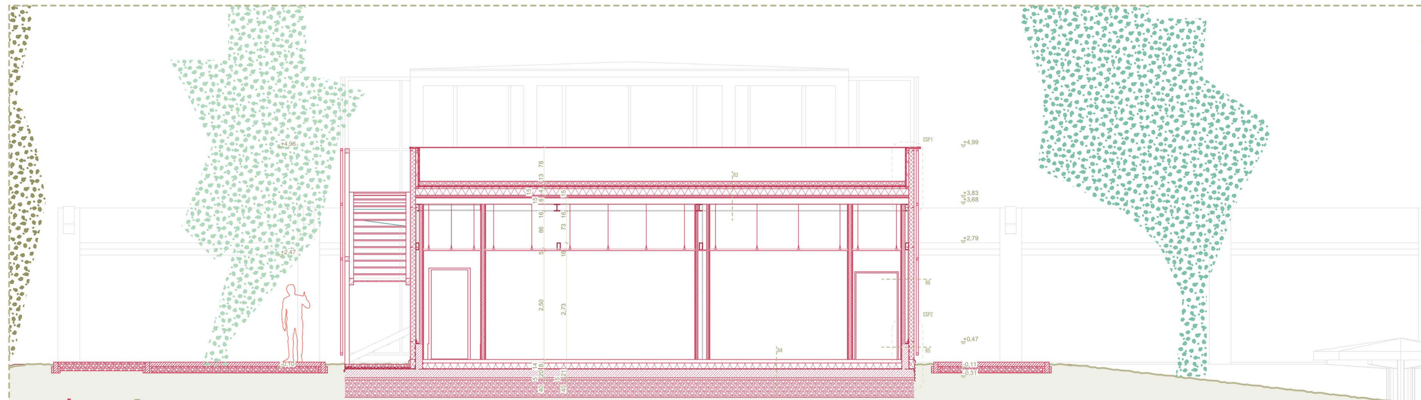
Főépület metszet 1:50
