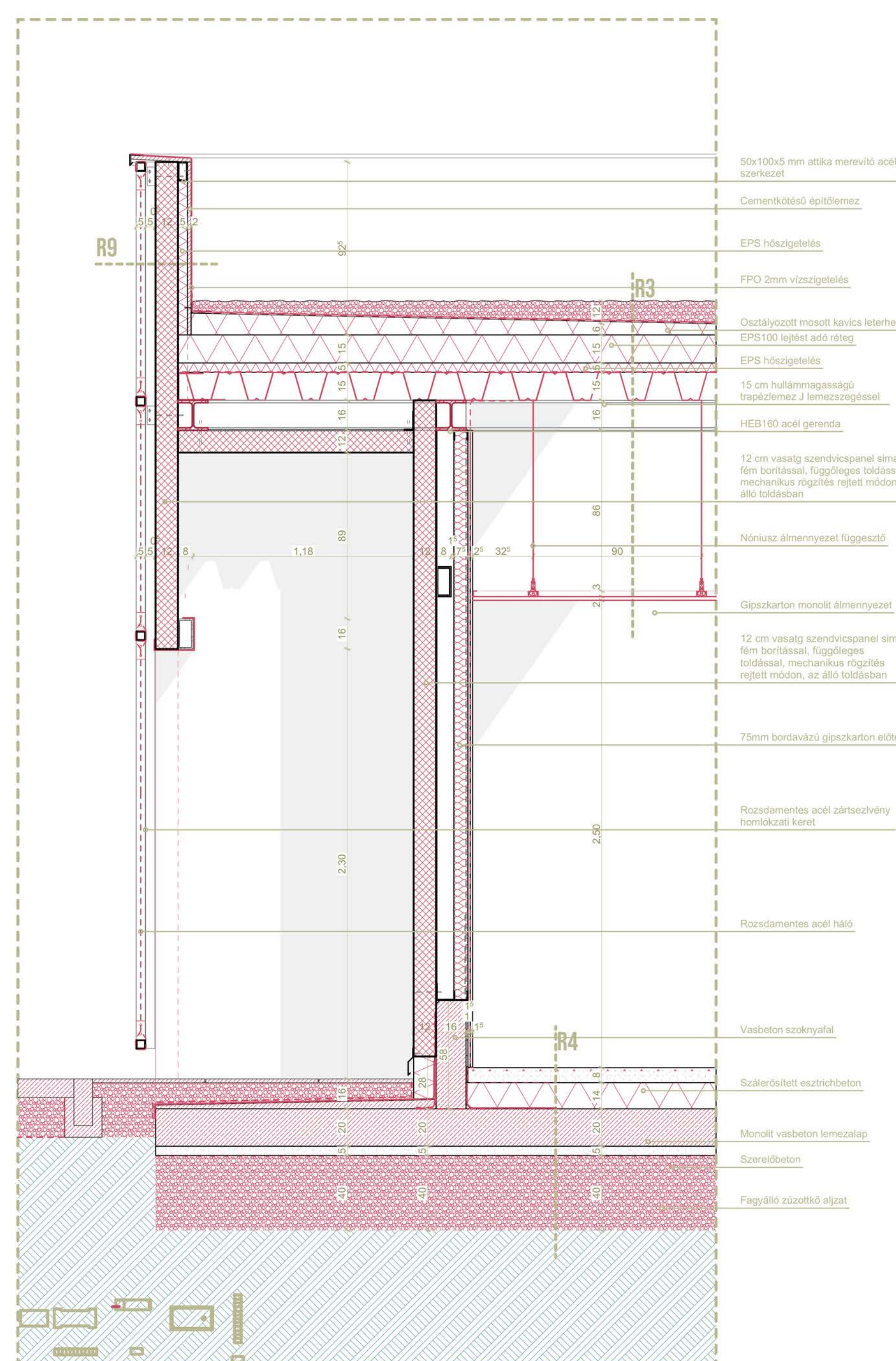
Főépület részmetset 1:20
