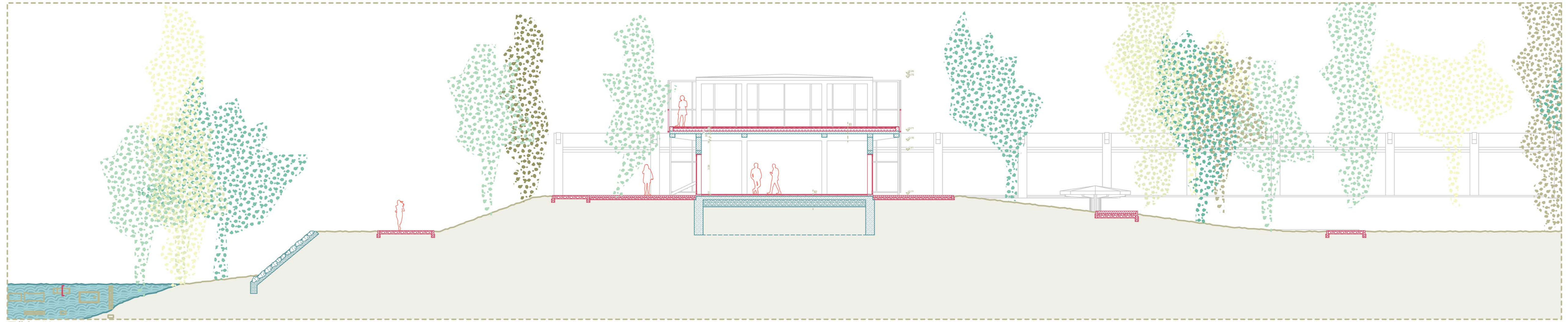
Főépület metszet 1:100
