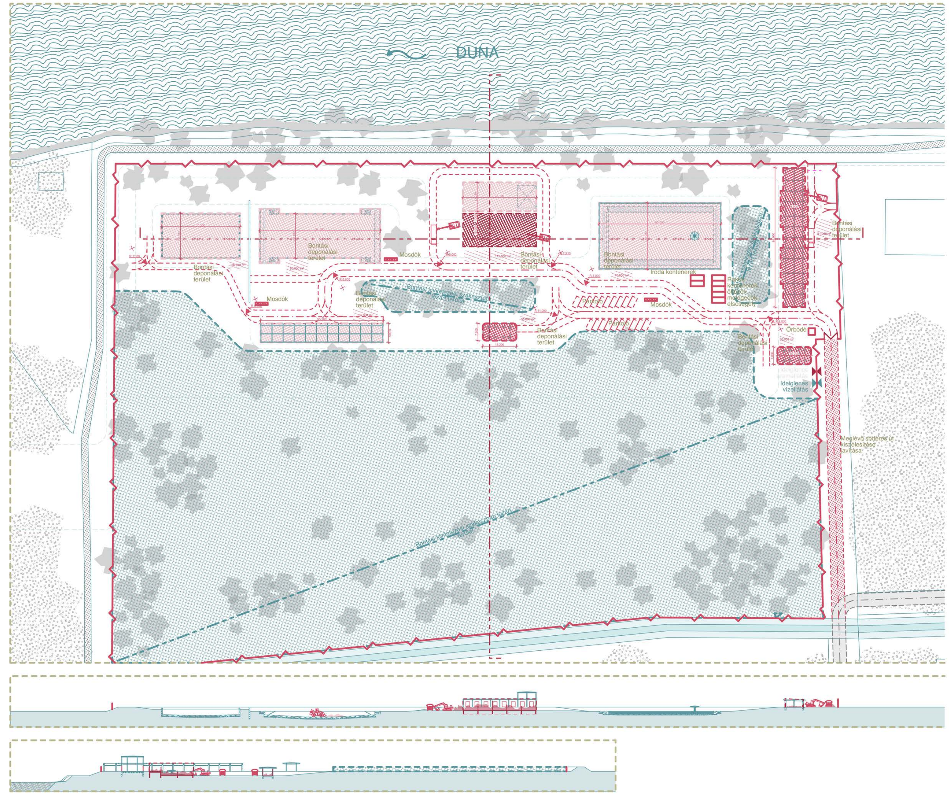
Bontási organizáció helyszínrajz 1:1000
