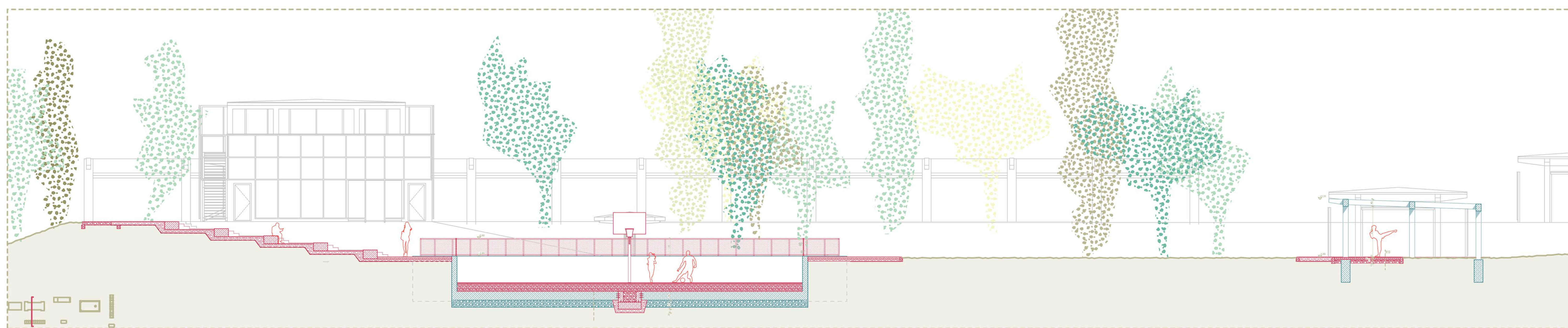
Sportpálya metszet 1:100
