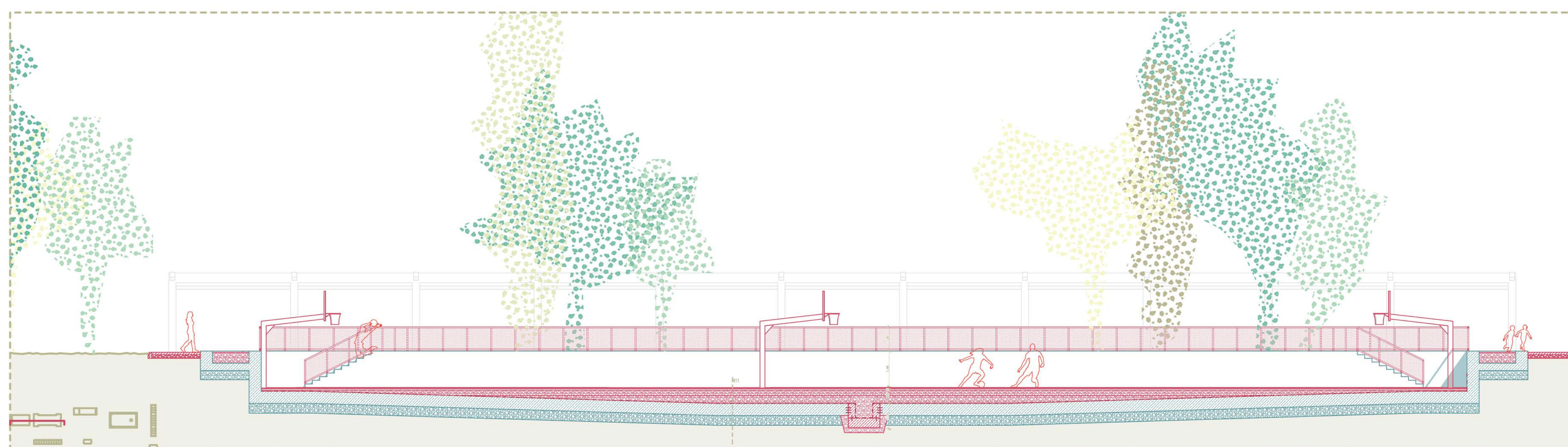
Sportpálya metszet 1:100
