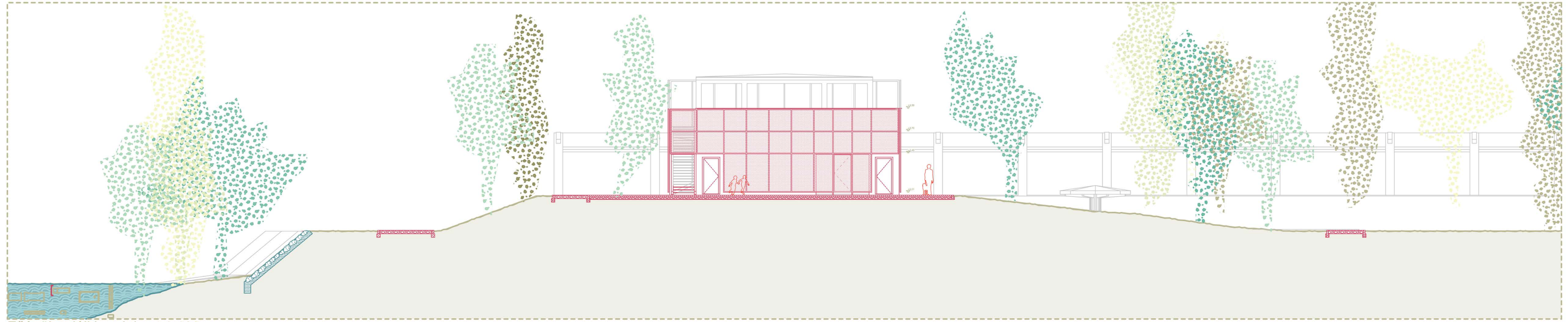
Főépület déli homlokzat 1:100
