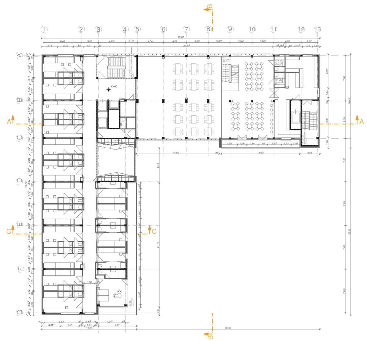
Első emeleti alaprajz m = 1 : 200
