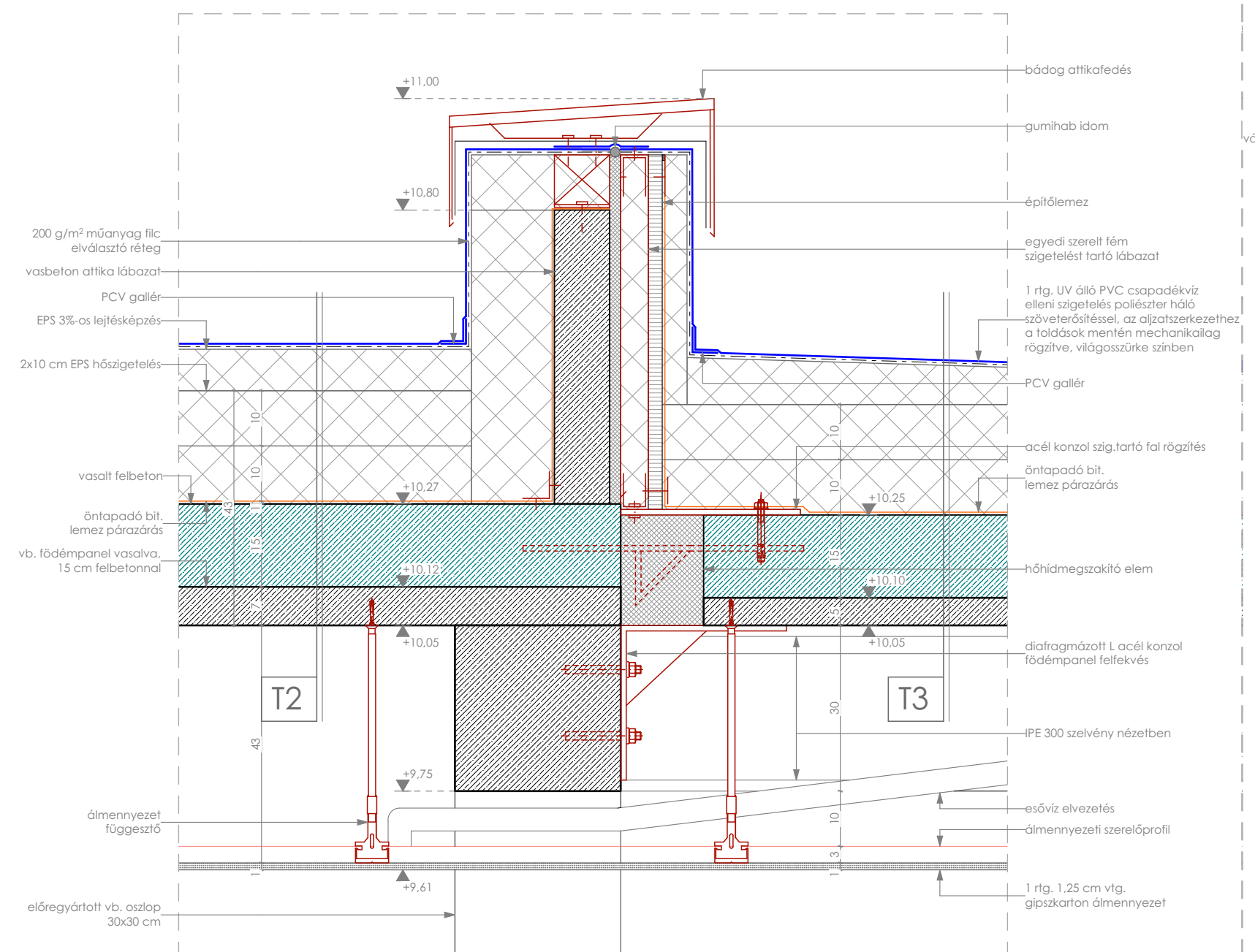
átkötőhid attika csomópont M=1:10
