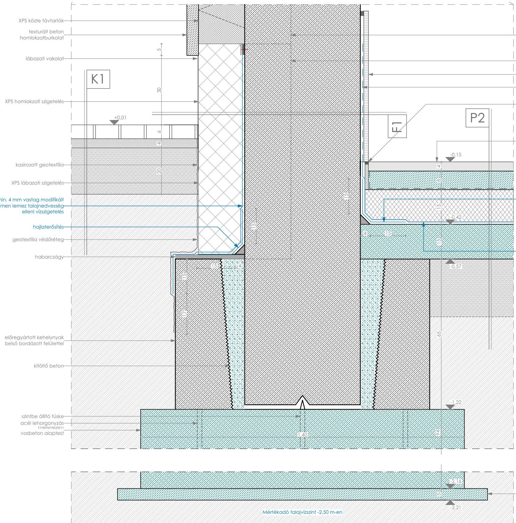
kehelyalap csomópont M=1:10
