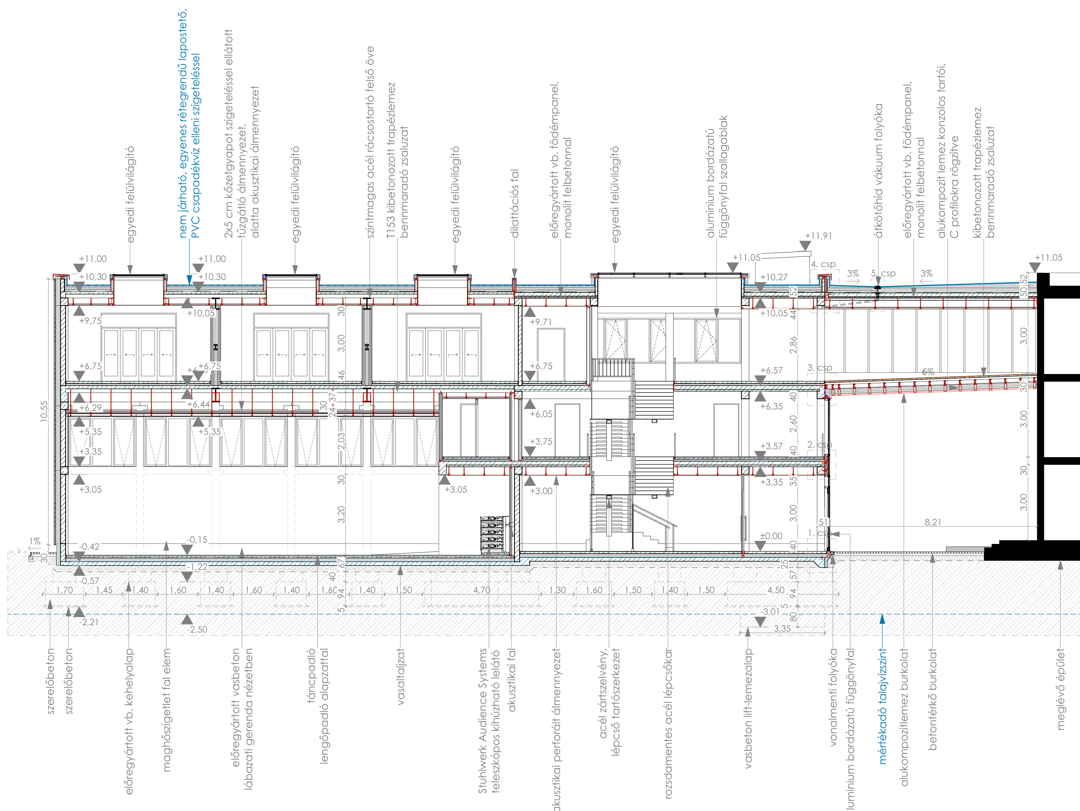
A metszet
