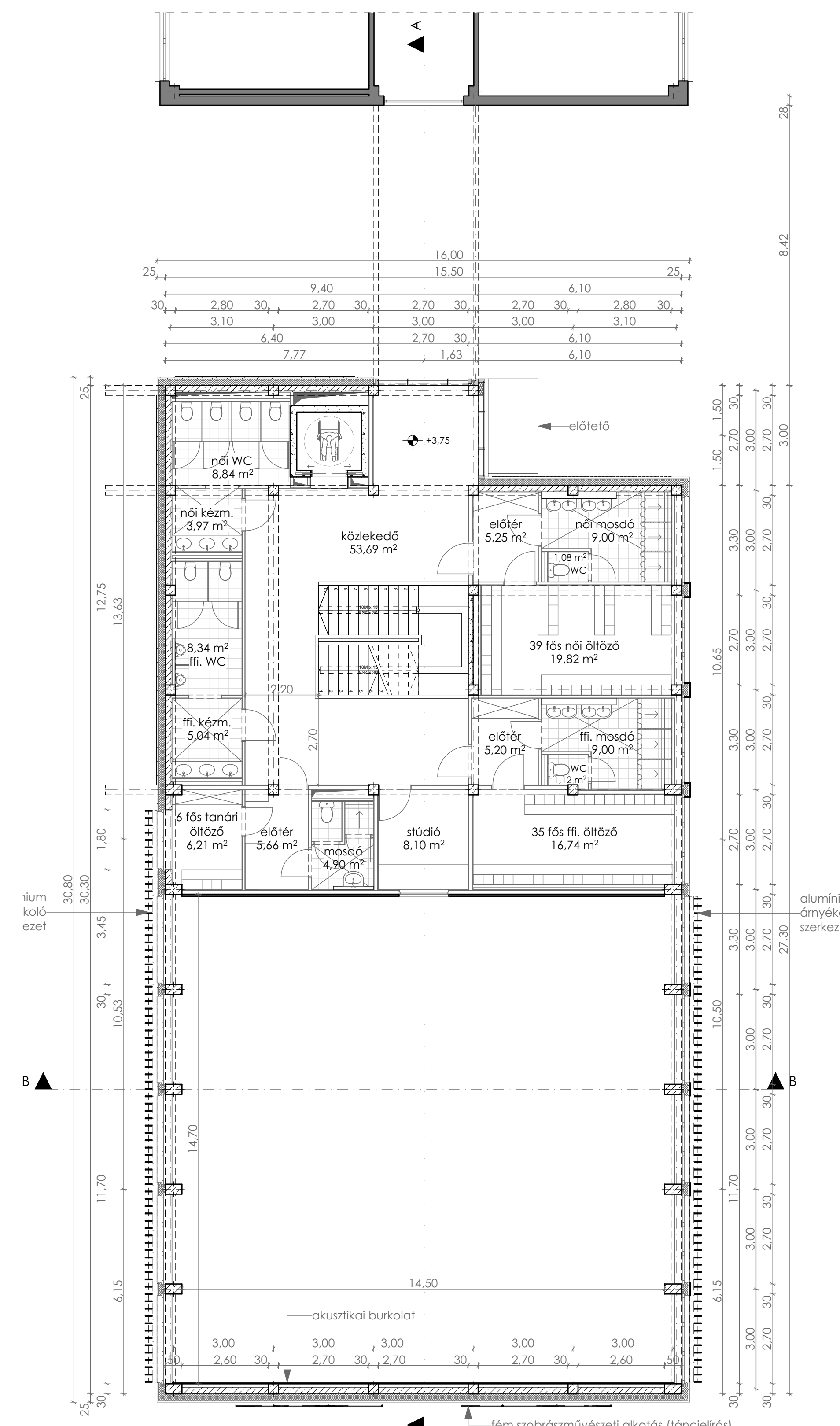
1. emeleti alaprajz M=1:100
