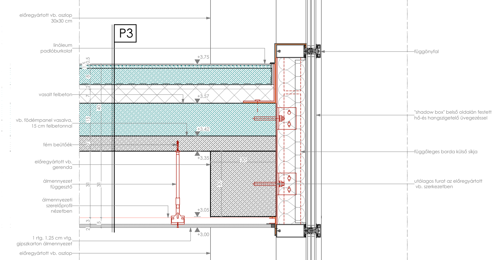
szintközi függőnyfal csomópont M=1:10
