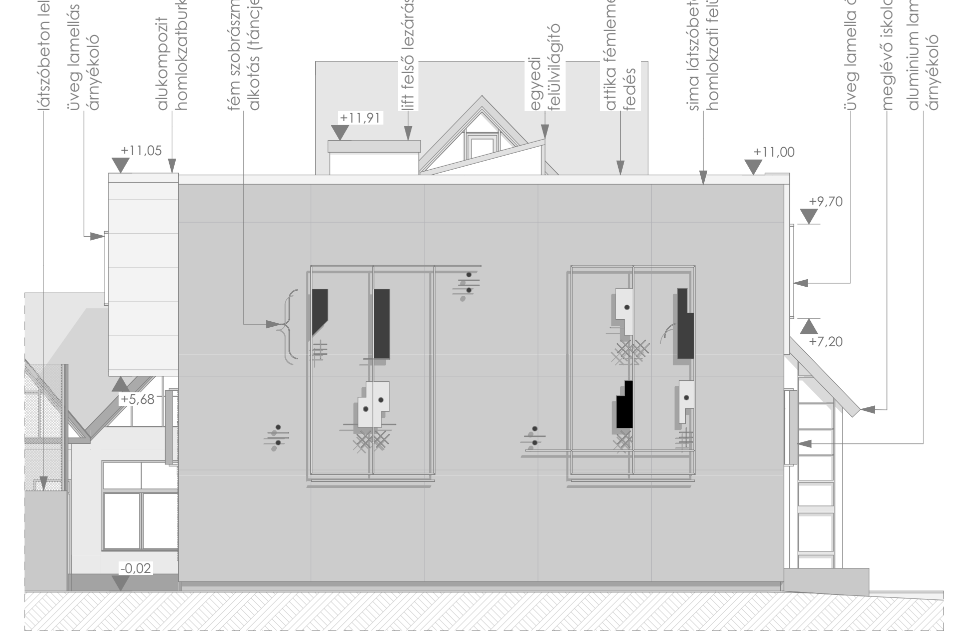
D homlokzat M=1:100
