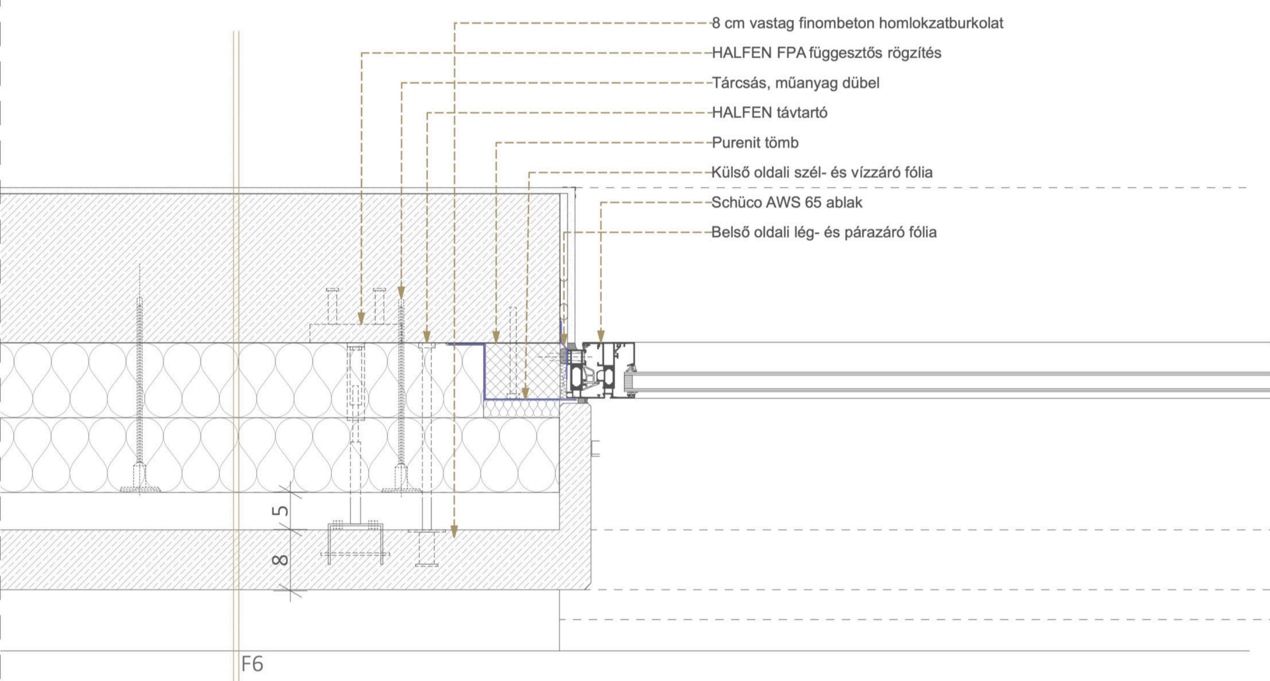
11. CSOMÓPONT M=1:5
