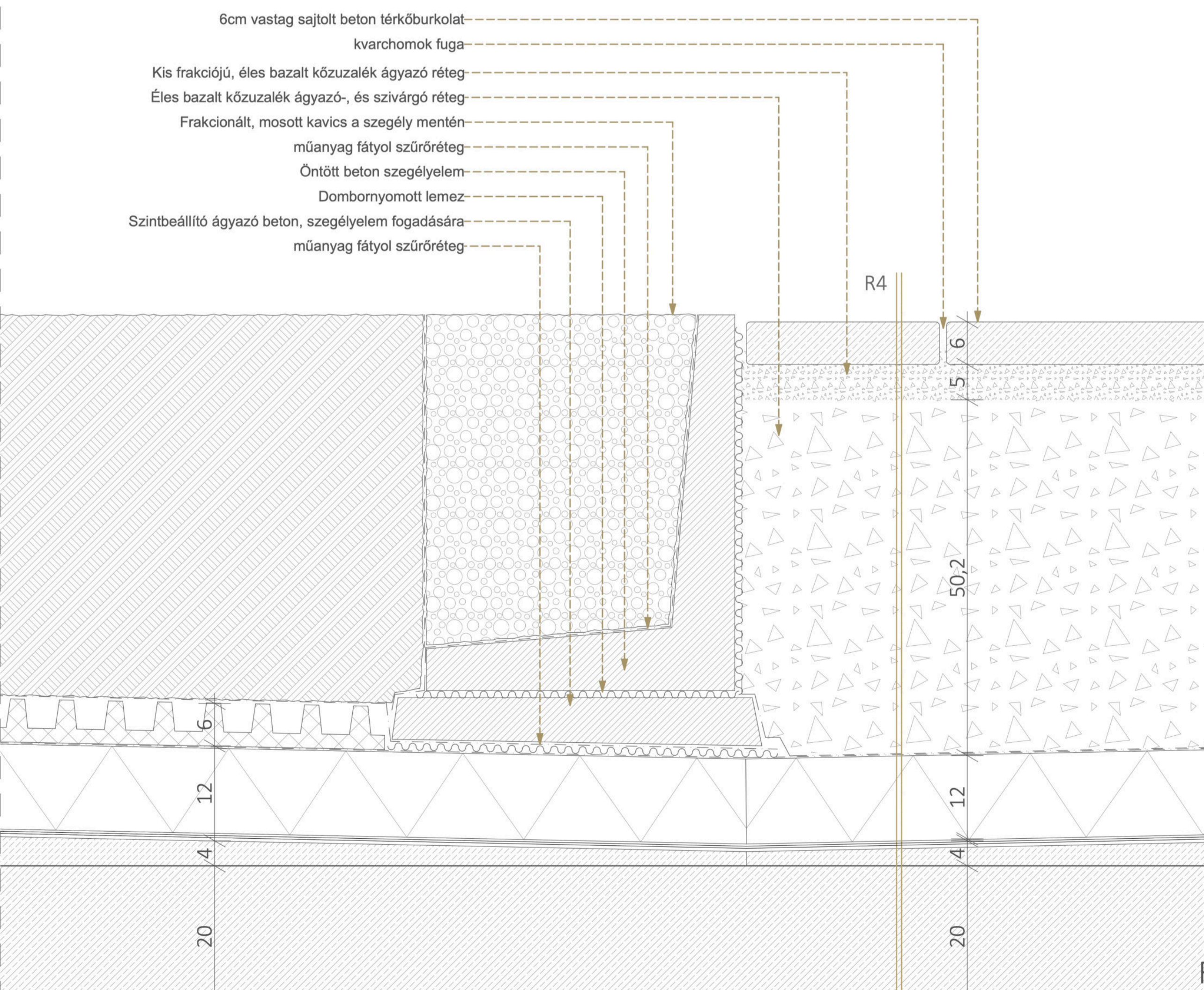
12. CSOMÓPONT M=1:5
