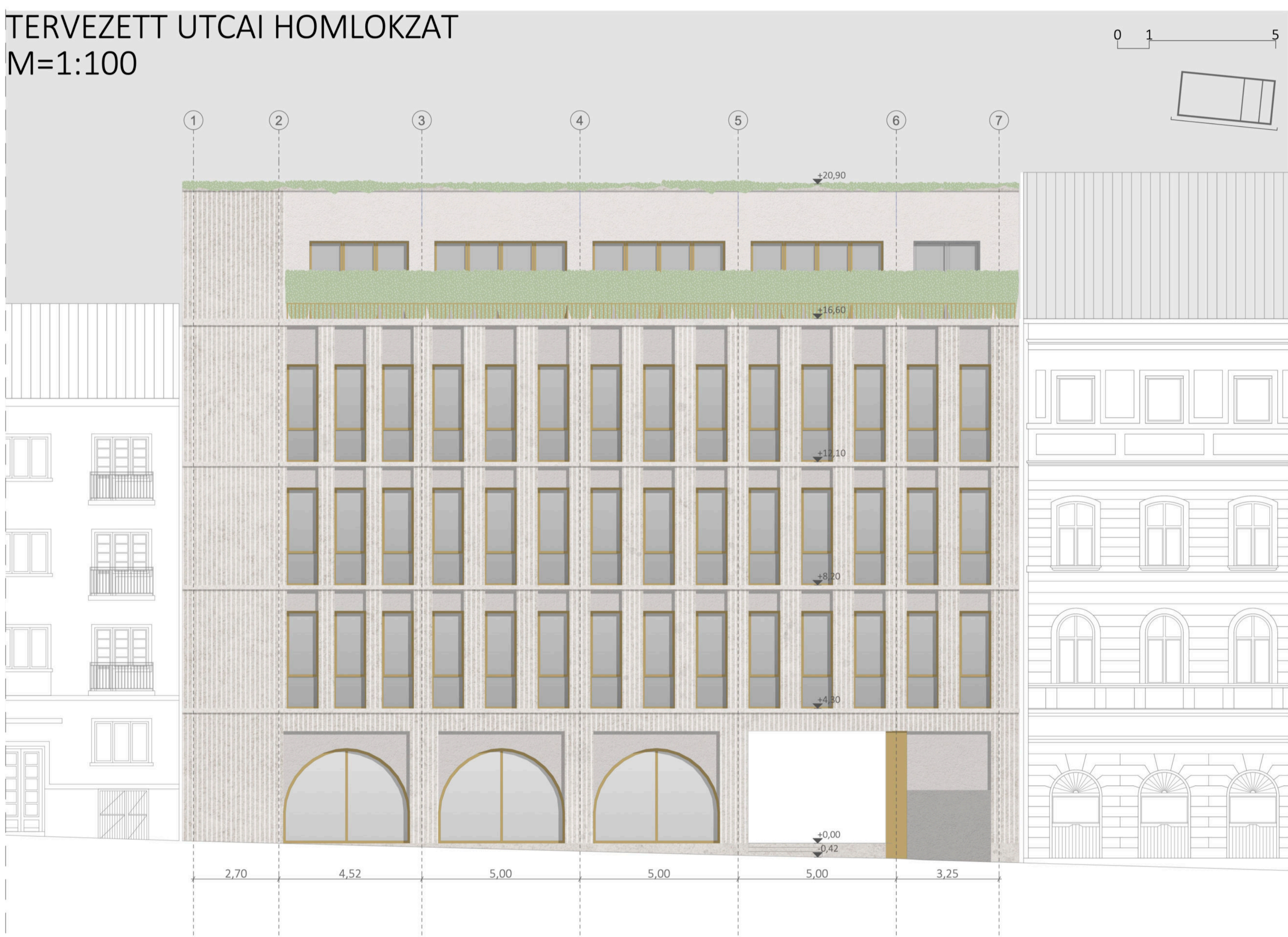
TERVEZETT UDVARI HOMLOKZAT M=1:100
