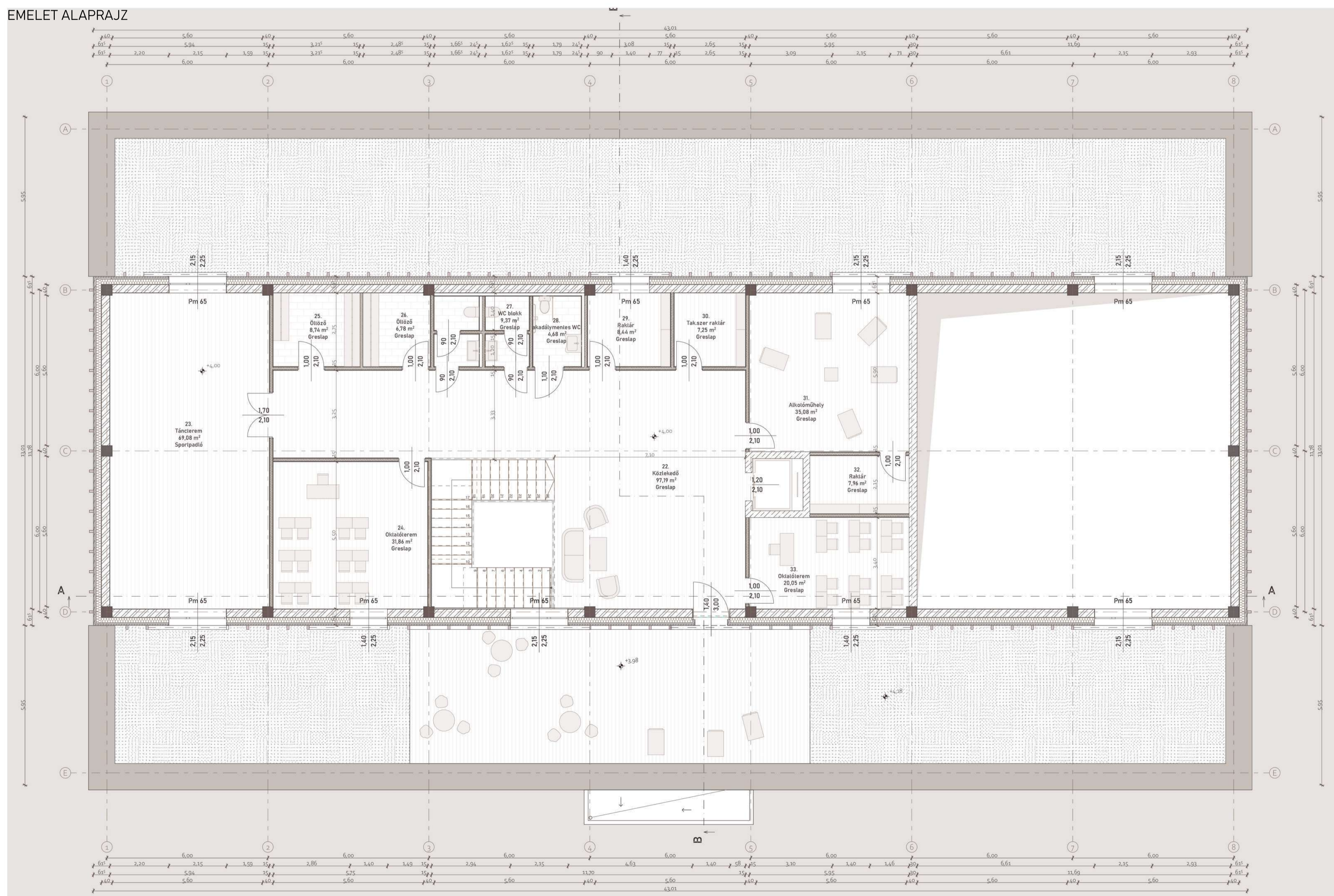
EMELET ALAPRAJZ
