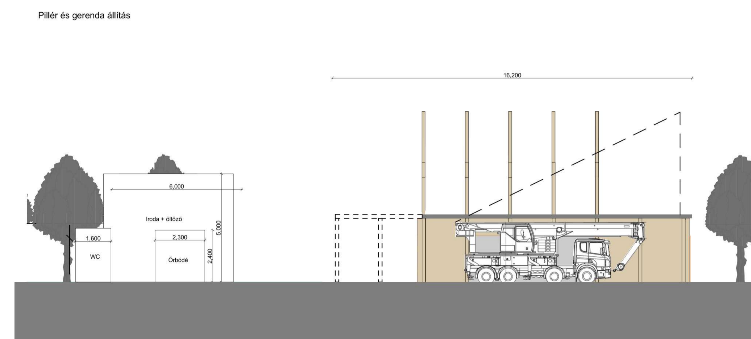
ORGANIZÁCIÓ, GERENDA ÉS PILLÉR ÁLLÍTÁS M=1:100
