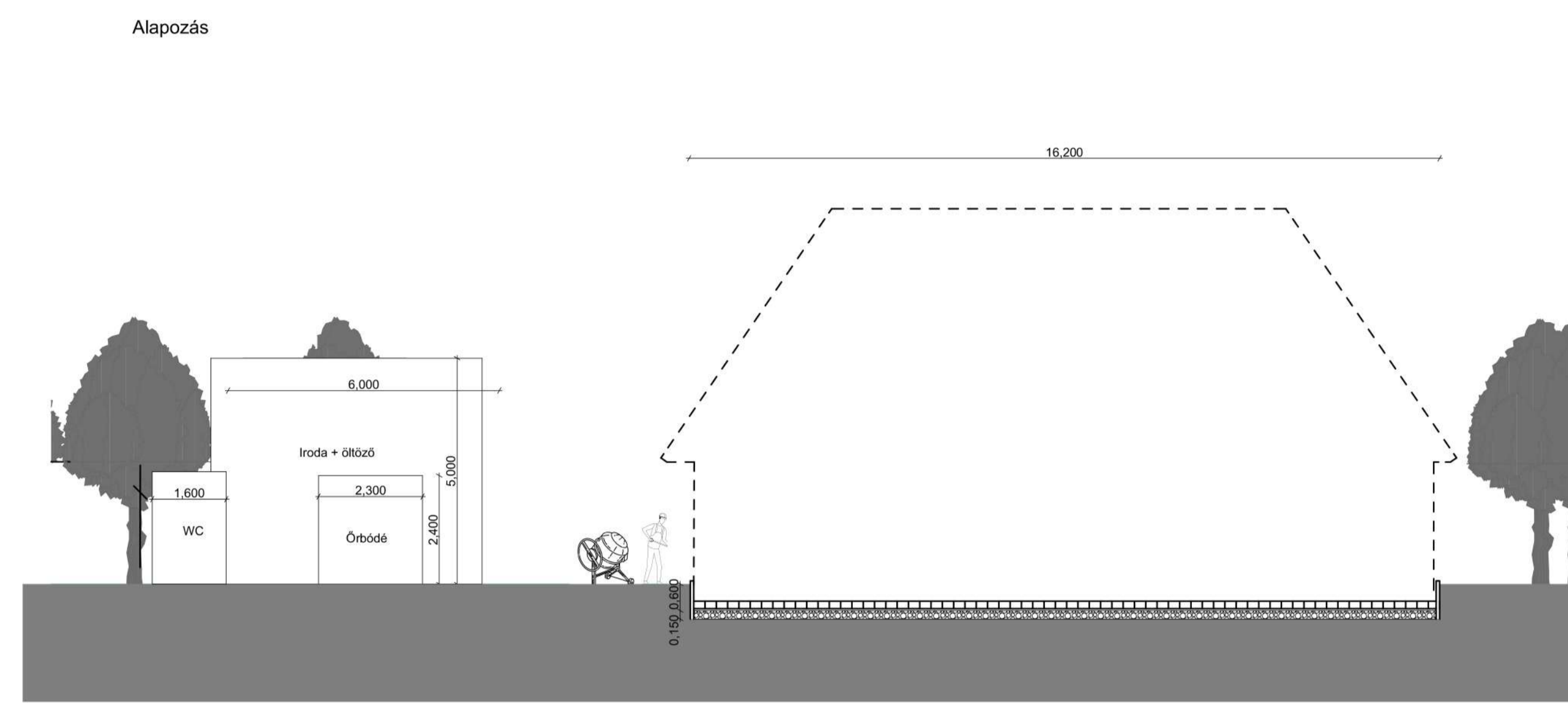
ORGANIZÁCIÓ, ALAPOZÁS M=1:100
