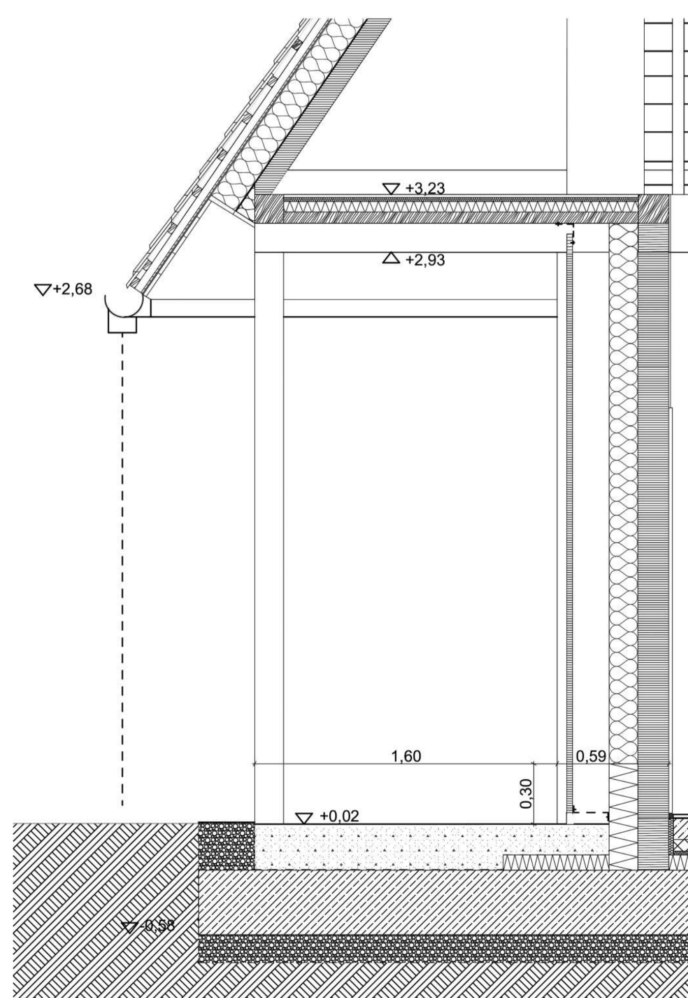
METSZET RÉSZLET M=1:20
