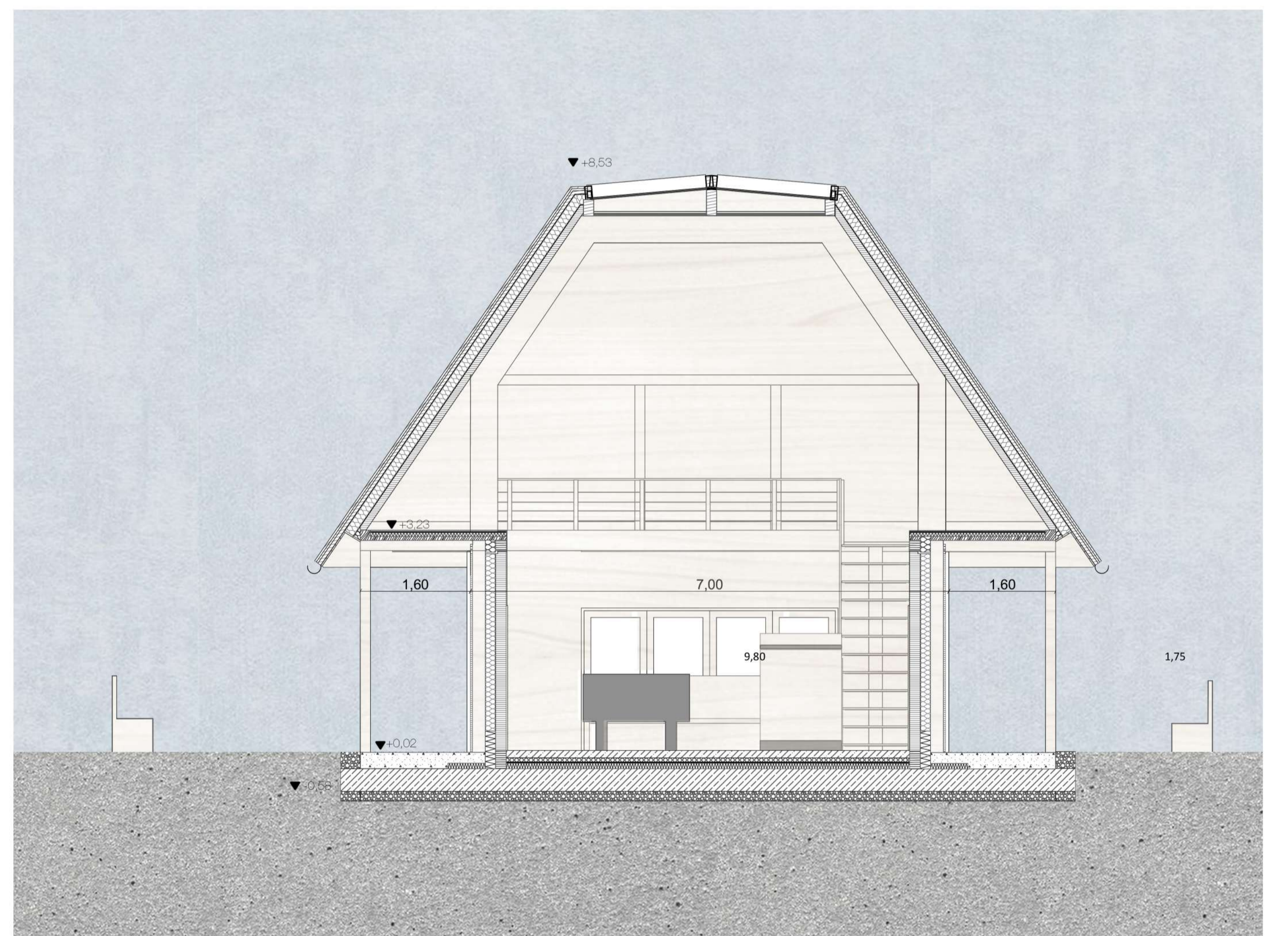
METSZET M=1:50
