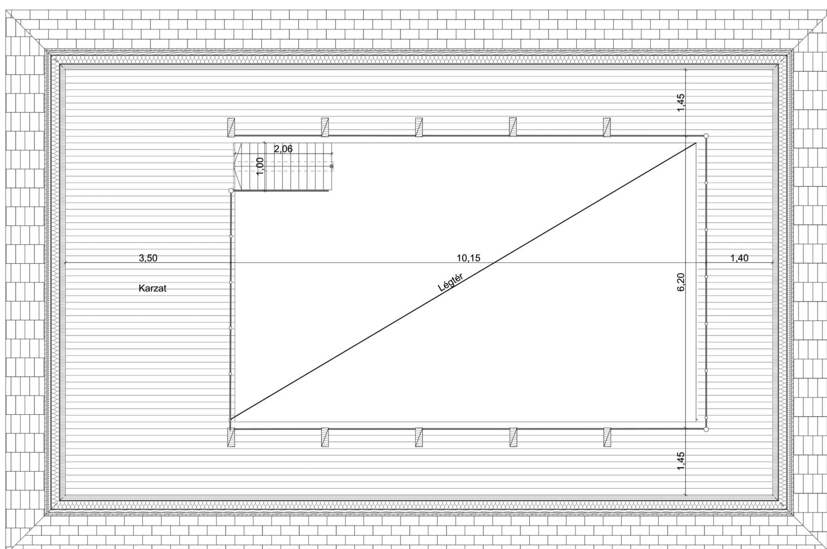
ALAPRAJZ KARZAT M=1:50
