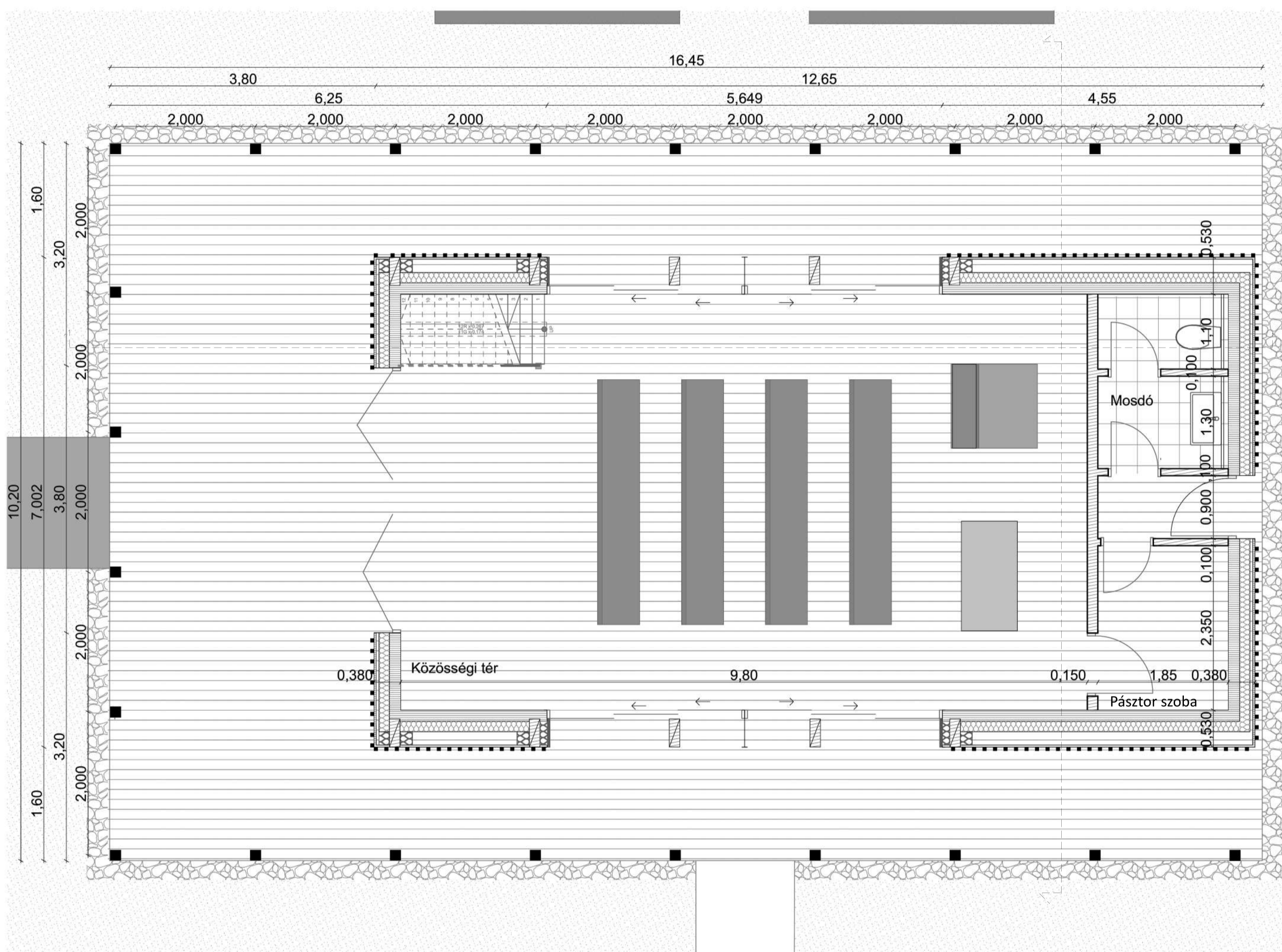
ALAPRAJZ FÖLDSZINT M=1:50
