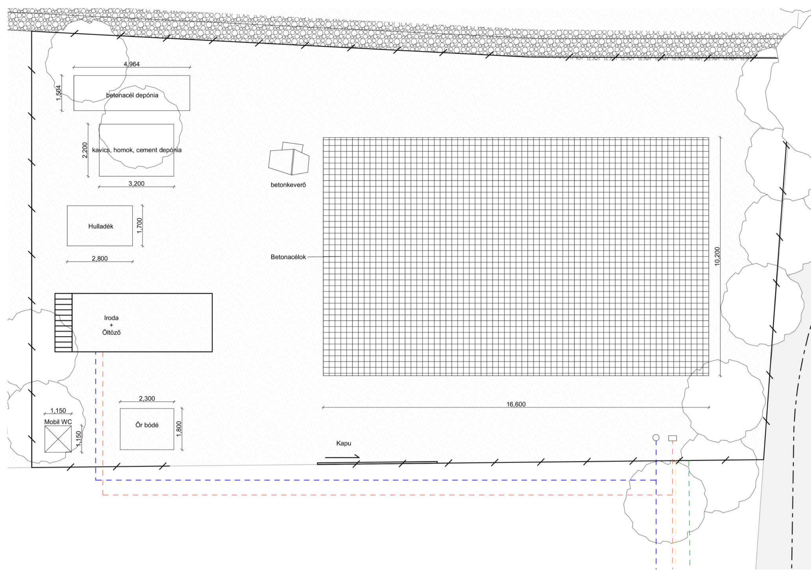
ORGANIZÁCIÓ, ALAPOZÁS M=1:100
