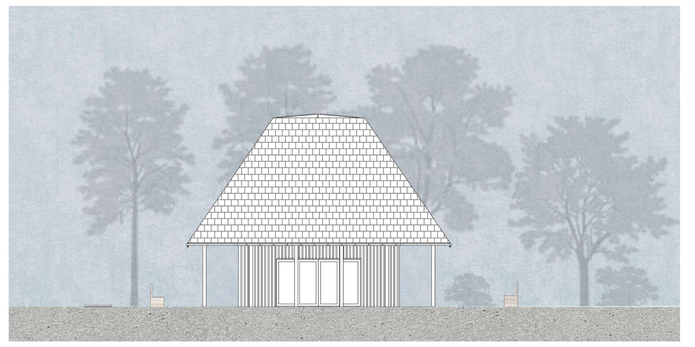
HOMLOKZAT NYUGAT M=100
