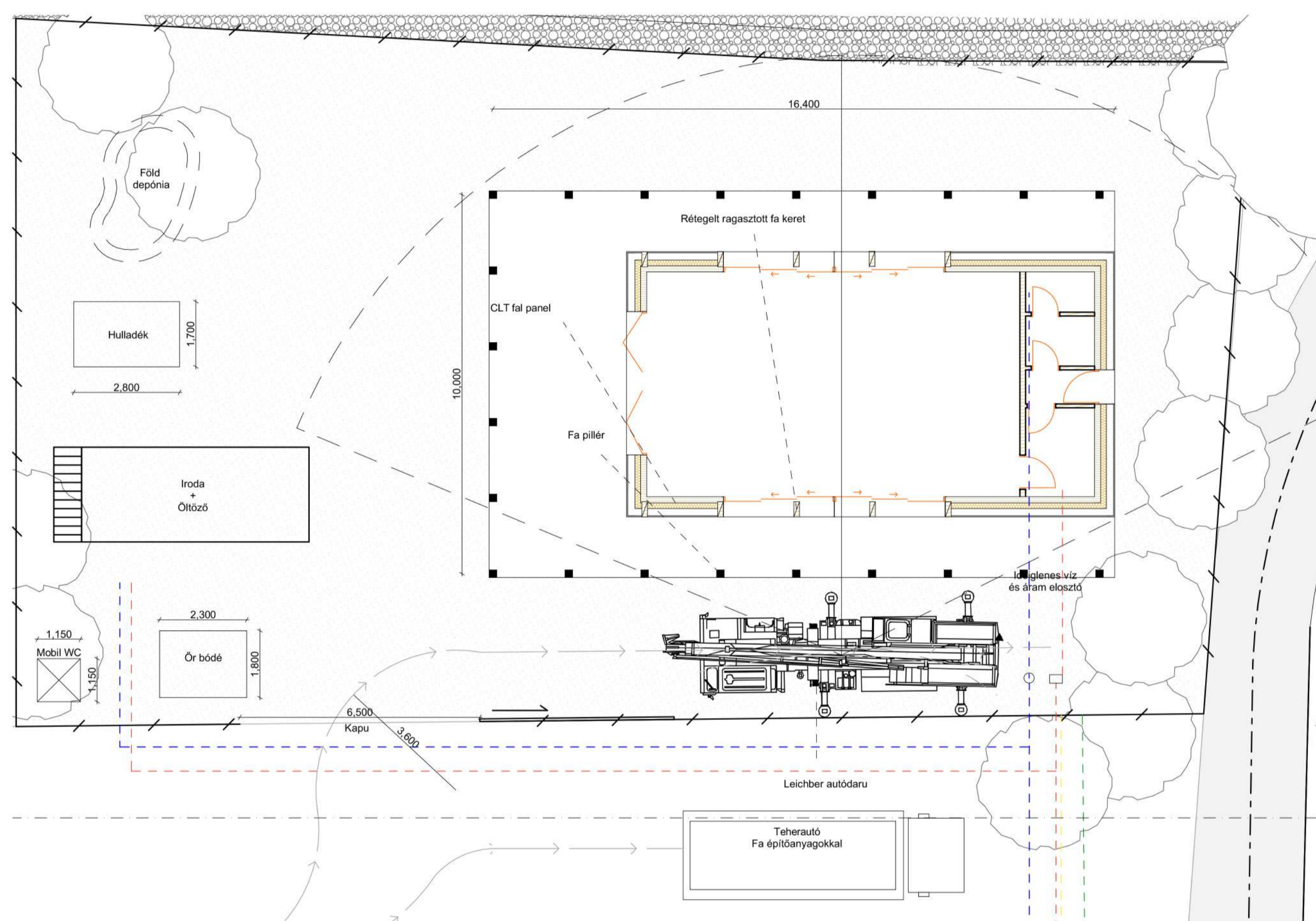
ORGANIZÁCIÓ, GERENDA ÉS PILLÉR ÁLLÍTÁS M=1:100
