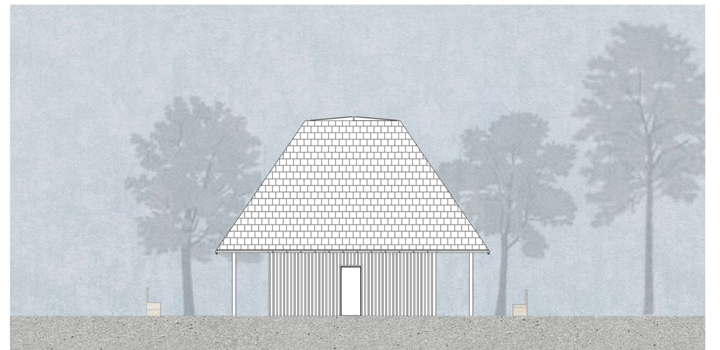
HOMLOKZAT KELET M=1:100
