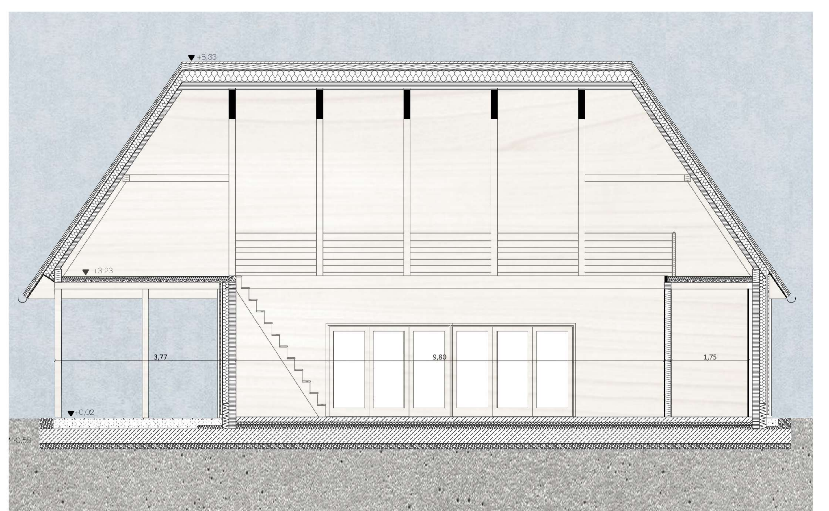
METSZET M=1:50
