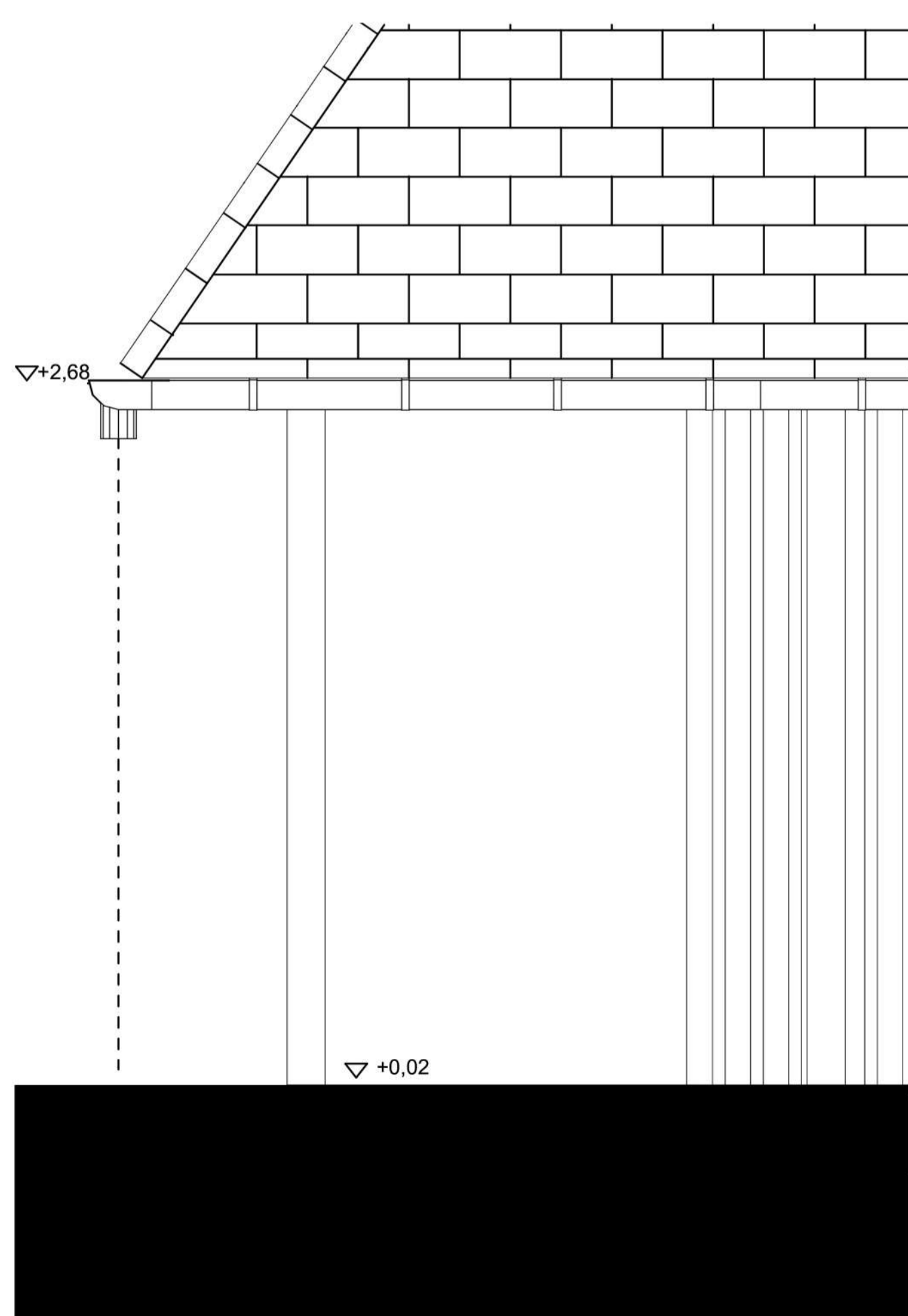
HOMLOKZATI RÉSZLET M=1:20
