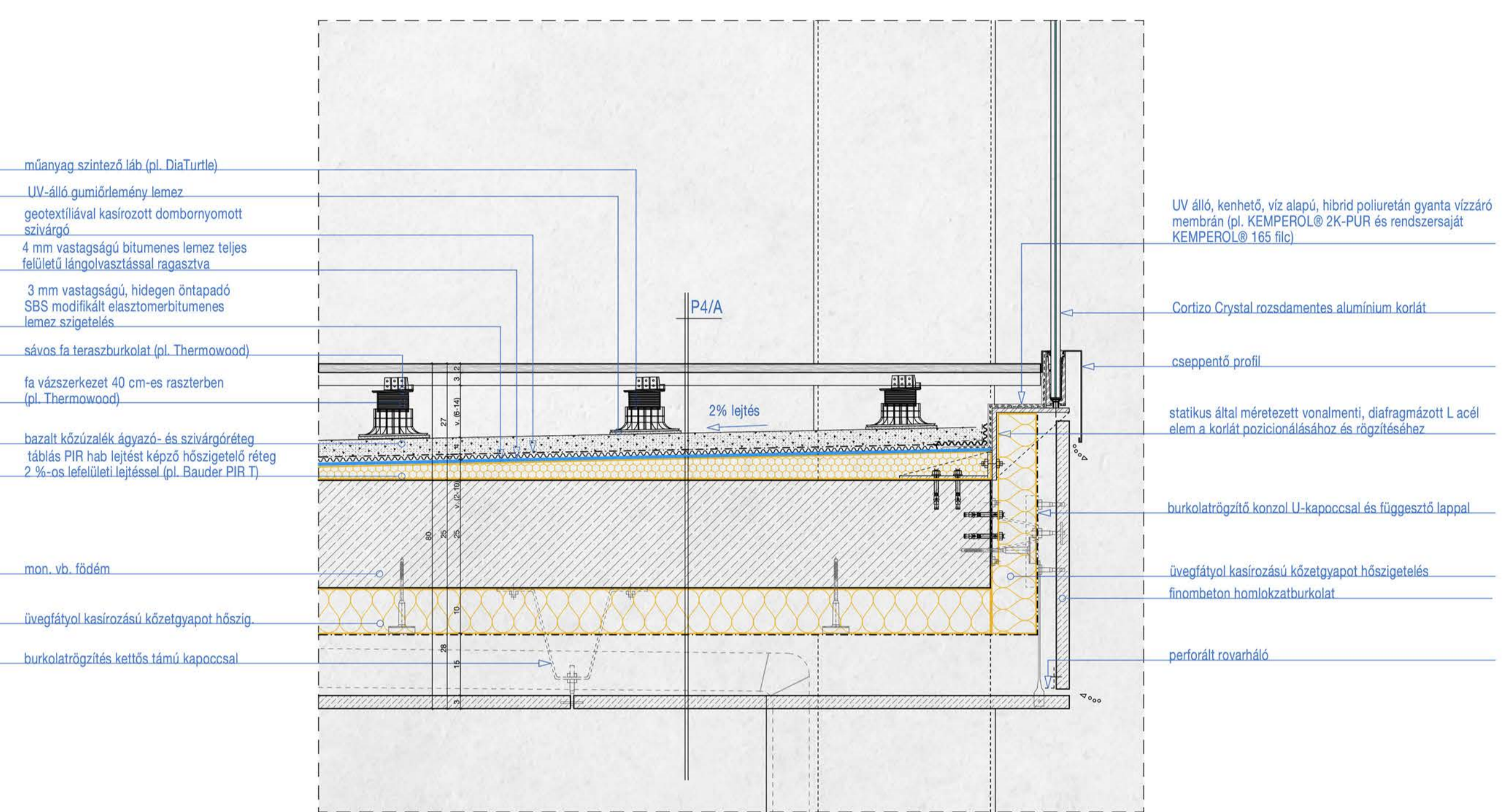
R08 RÉSZLETRAJZ - ÜVEGKORLÁT RÖGZÍTÉSE ERKÉLYPEREMEN M= 1:10
