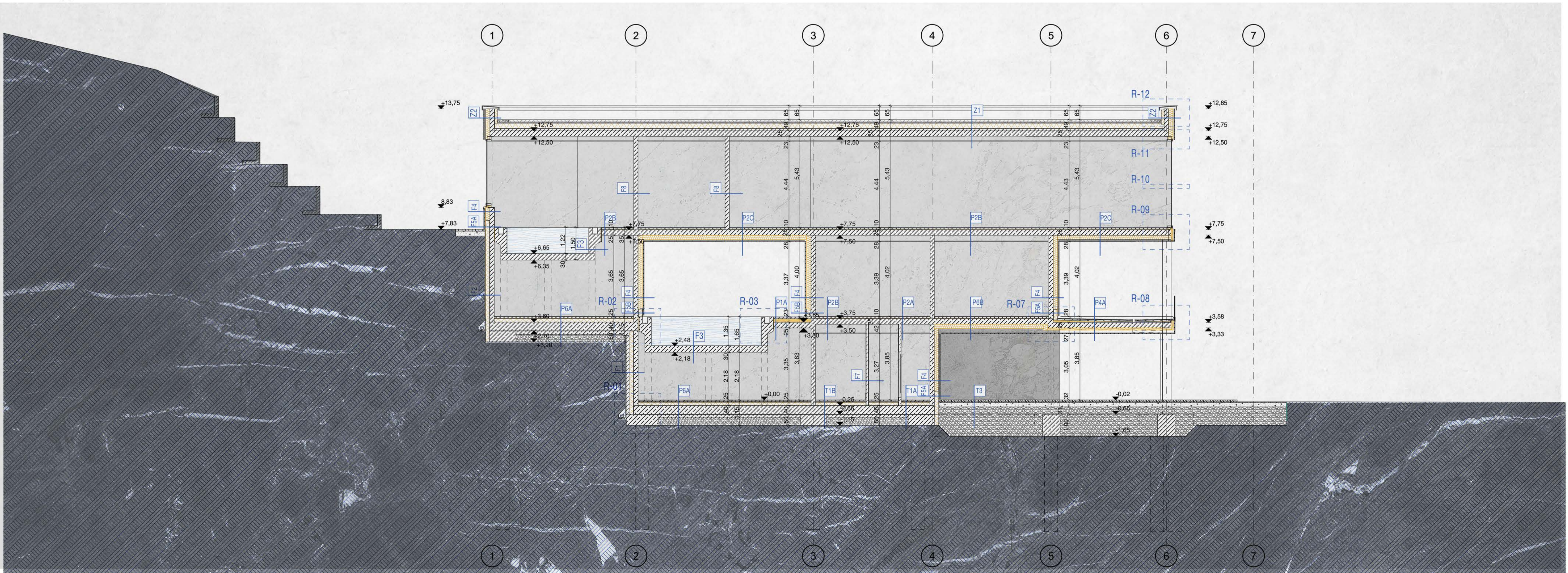
A-A METSZET M= 1:100
