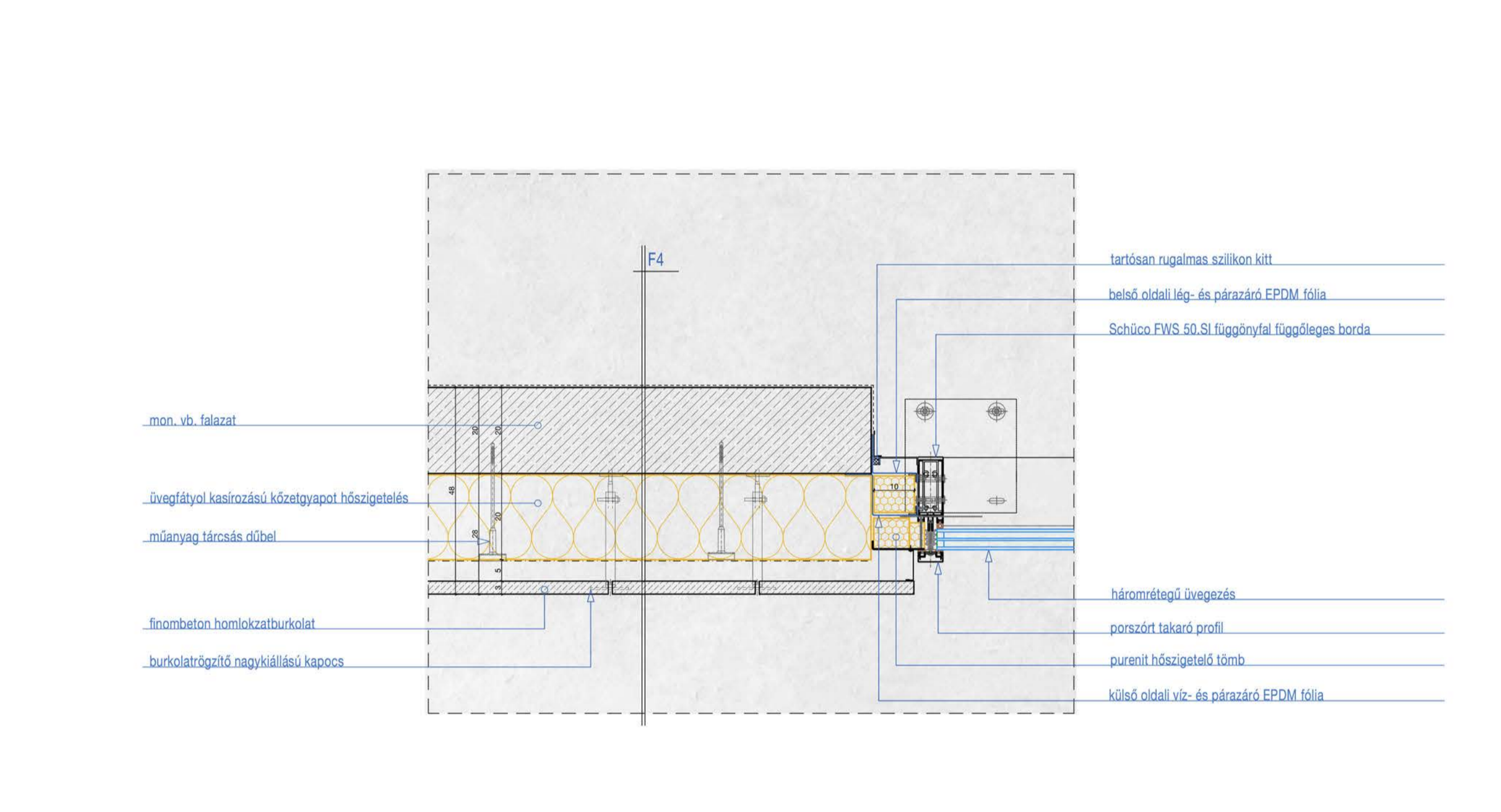
R09 RÉSZLETRAJZ - FÜGGÖNYFAL OLDALSÓ RÉSZLETE M= 1:10
