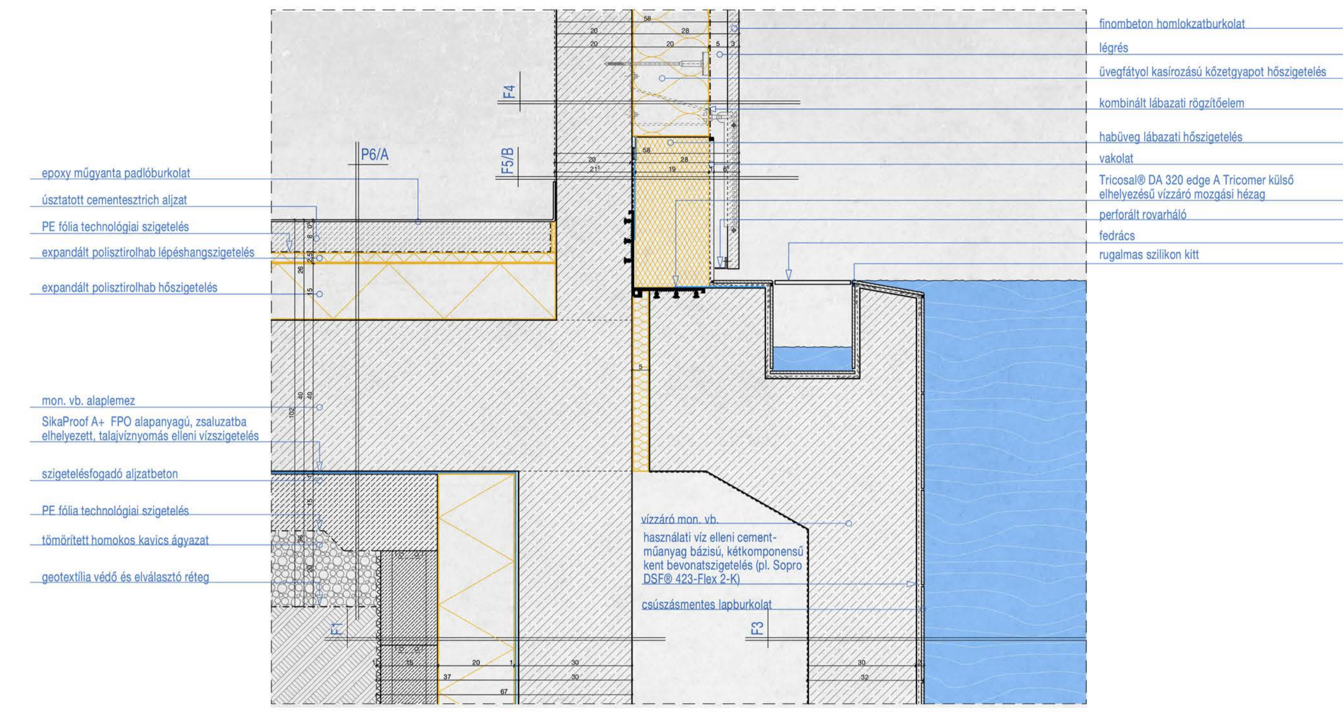
R02 RÉSZLETRAJZ - KÜLTÉRI MEDENCEPEREM SZINTUGRÁSÁNÁL M= 1:10
