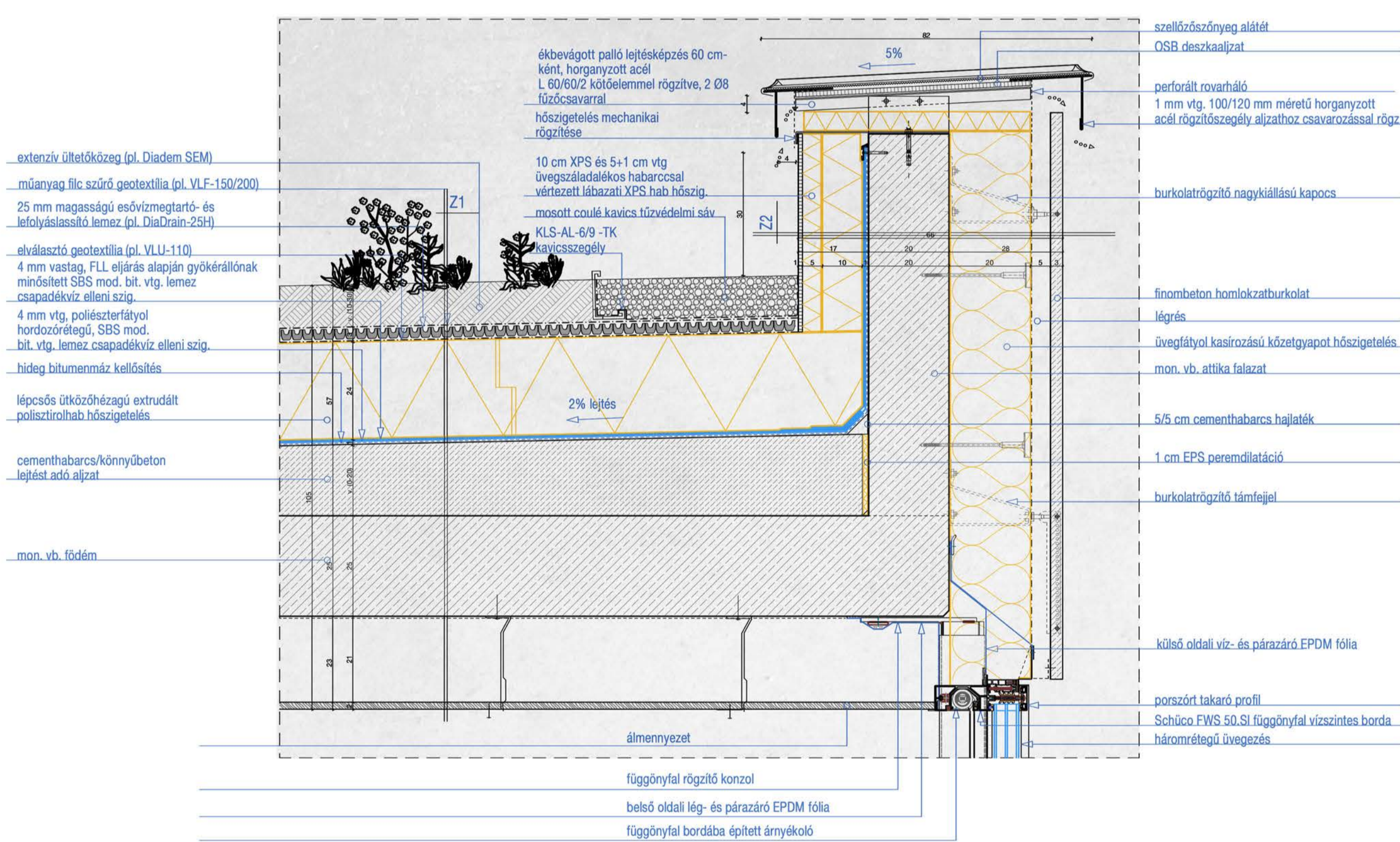
R11, R12 RÉSZLETRAJZ - FÜGGÖNYFAL FELSŐ ÉS ATTIKA KIALAKÍTÁS ZÁRÓFÖDÉMEN M= 1:10
