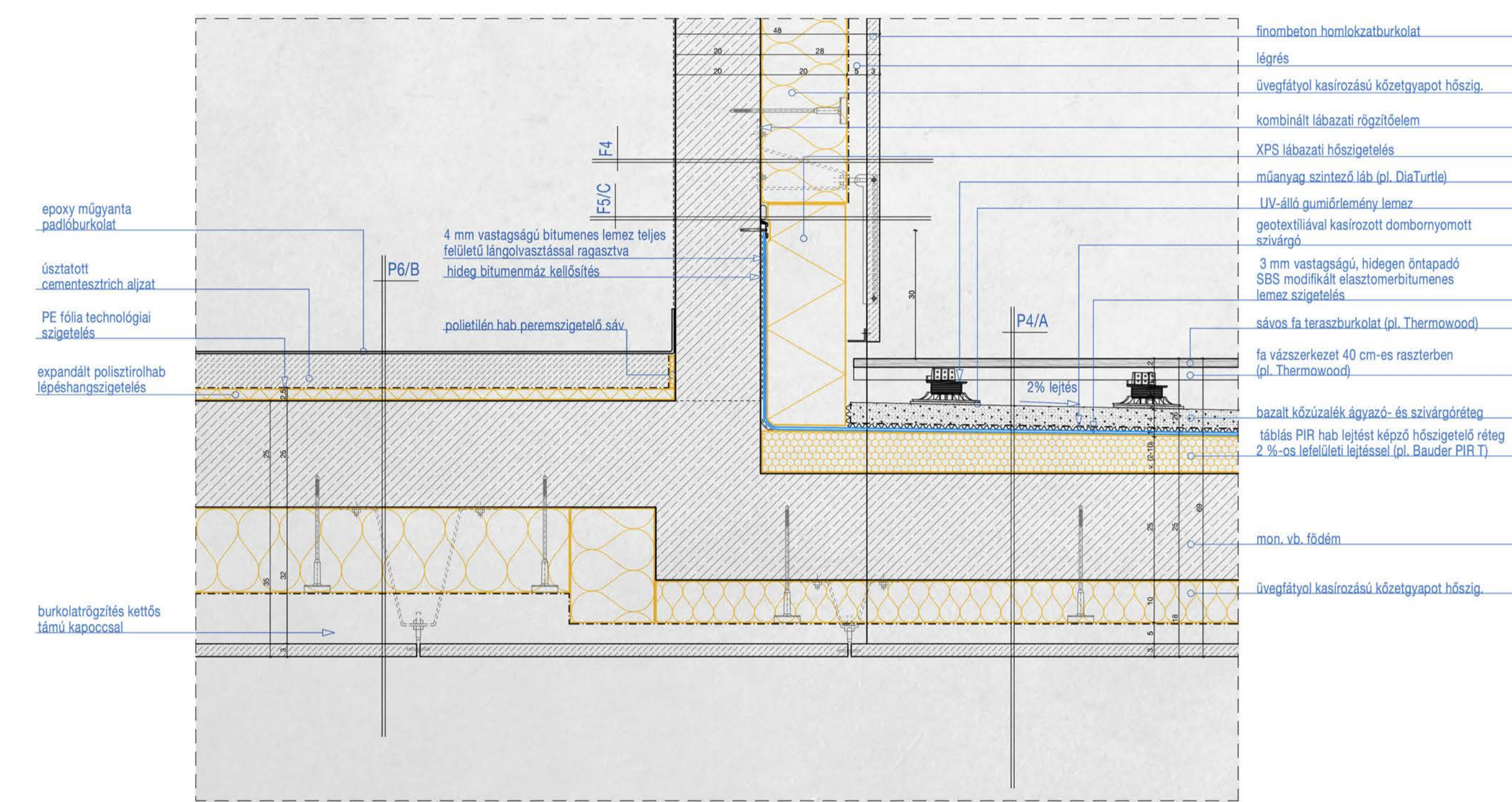
R07 RÉSZLETRAJZ - ÁLTALÁNOS LÁBAZATKÉPZÉS FÖDÉMUGRÁSÁNÁL, ERKÉLYEN M= 1:10
