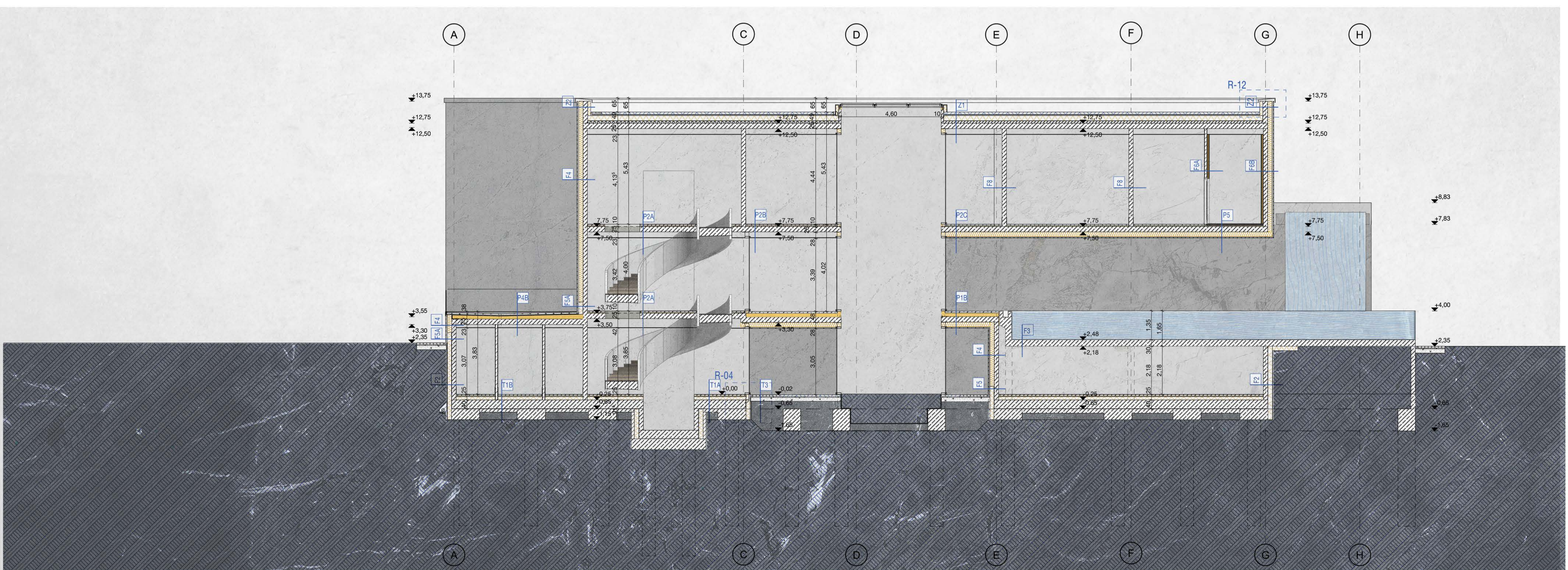
B-B METSZET M= 1:100
