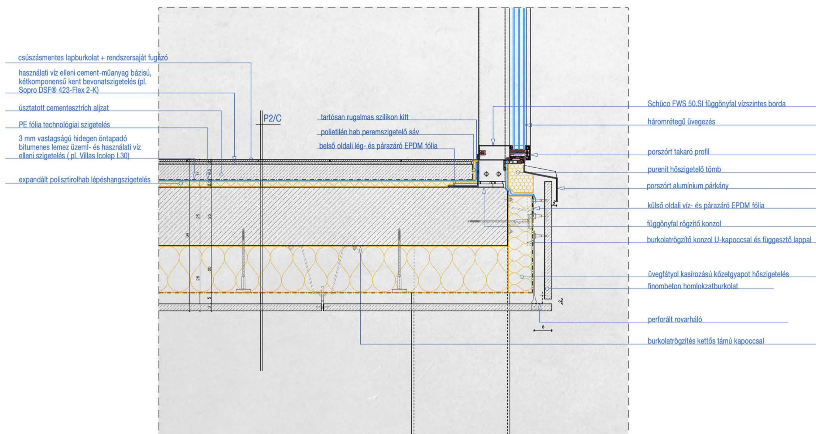
04 RÉSZLETRAJZ - FÜGGÖNYFAL LÁBAZATKIALAKÍTÁS FÖLDSZINTEN M= 1:10
