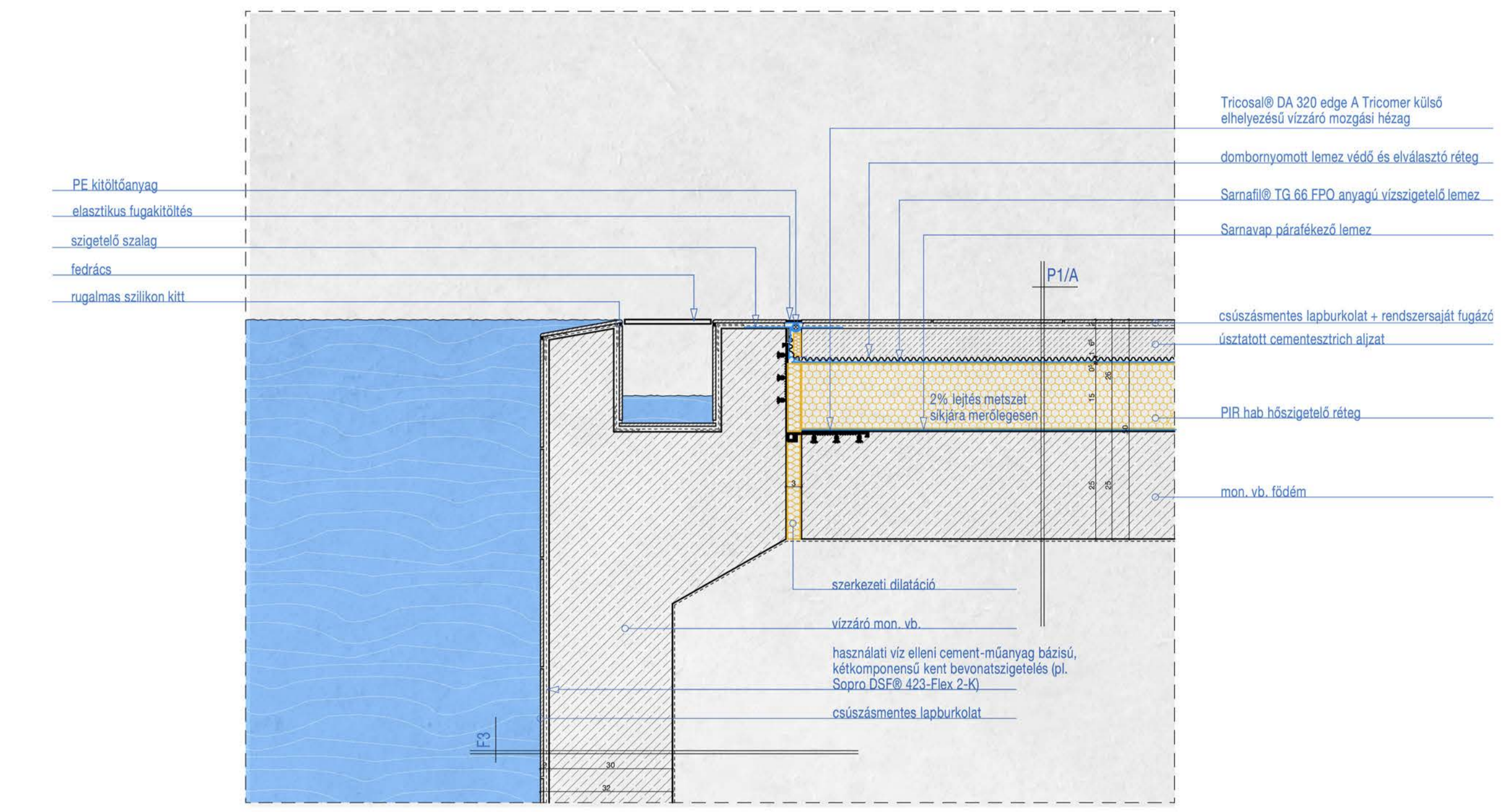
R03 RÉSZLETRAJZ - KÜLTÉRI MEDENCEPEREM LAPOSTETŐN M= 1:10
