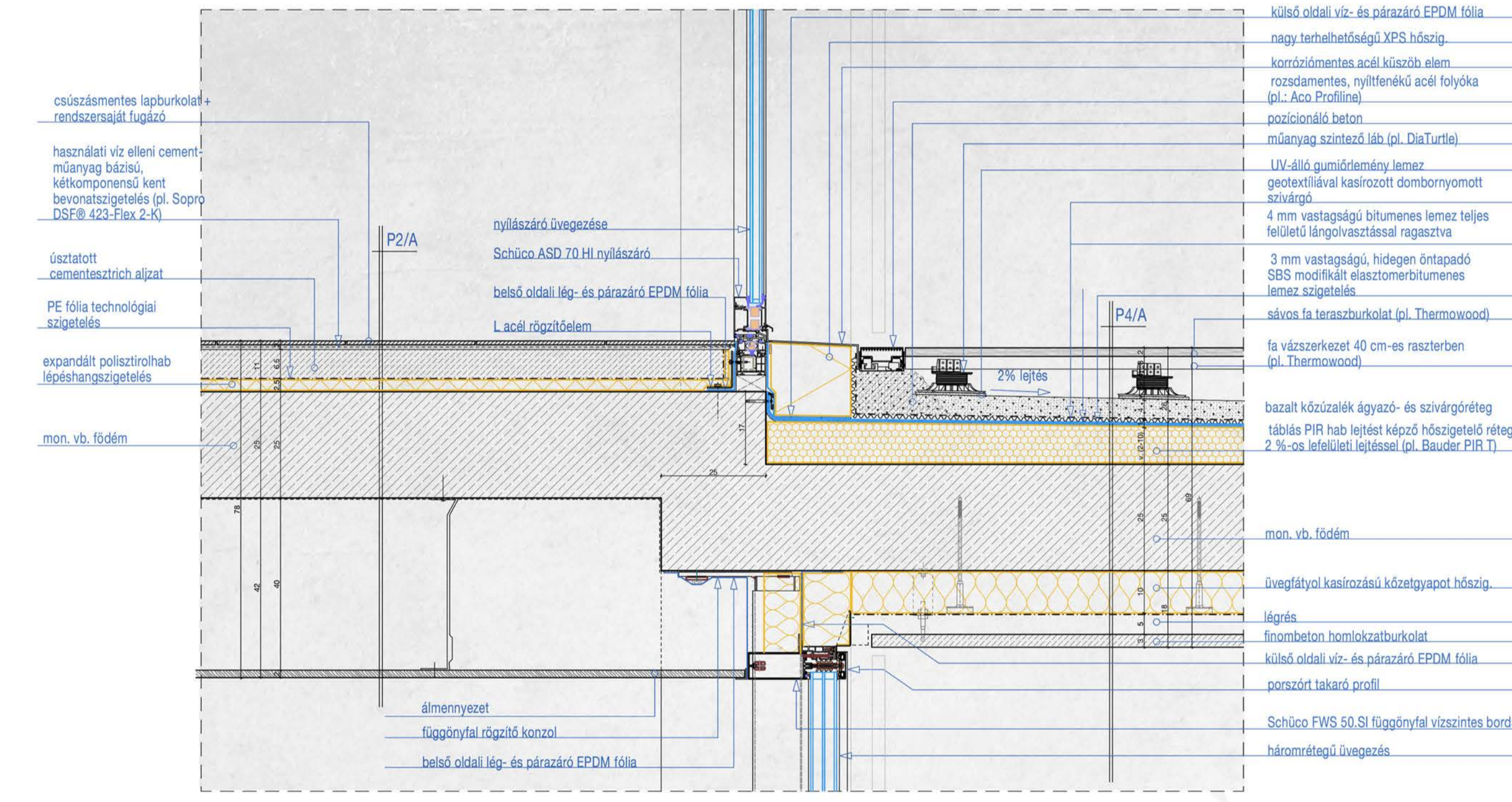
R05, R06 RÉSZLETRAJZ - TERASZAJTÓ KÜSZÖBKIALAKÍTÁS ÉS FÜGGÖNYFAL FELSŐ RÉSZLETE M= 1:10
