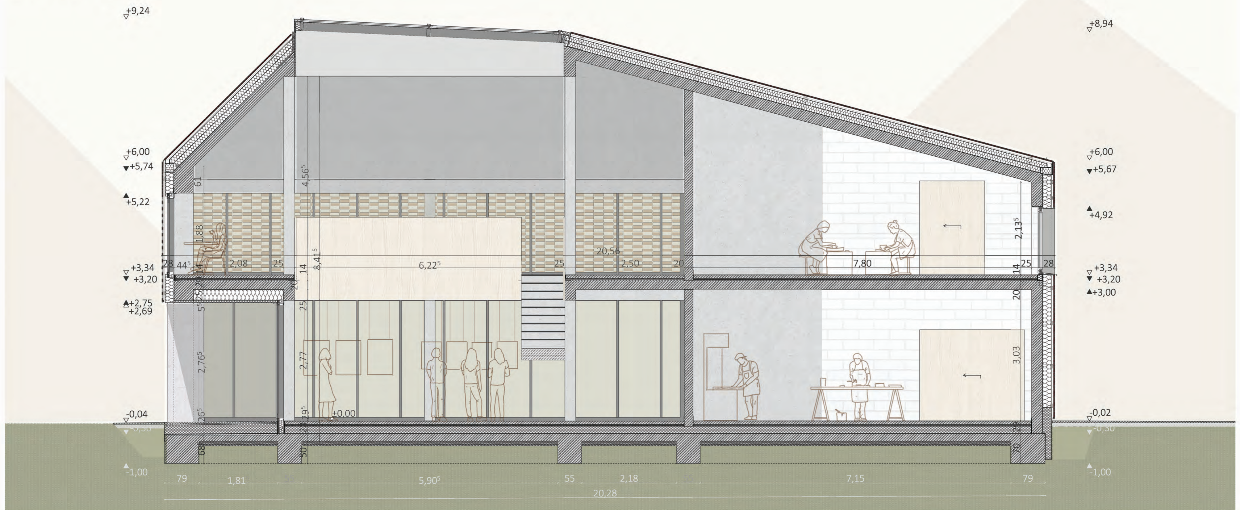
A METSZET 1:50
