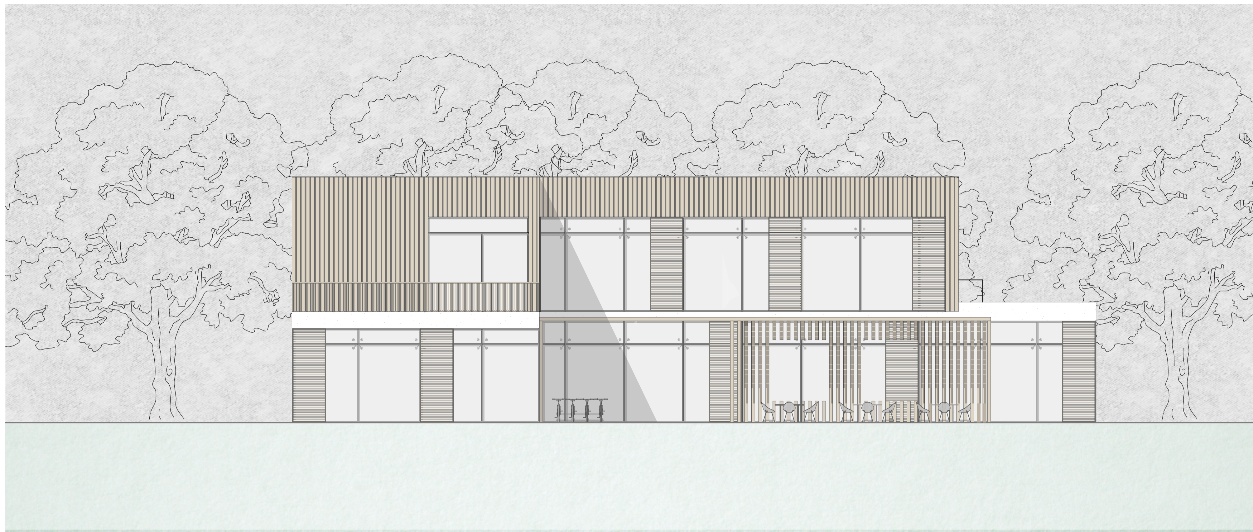
KELETI HOMLOKZAT M=1:100
