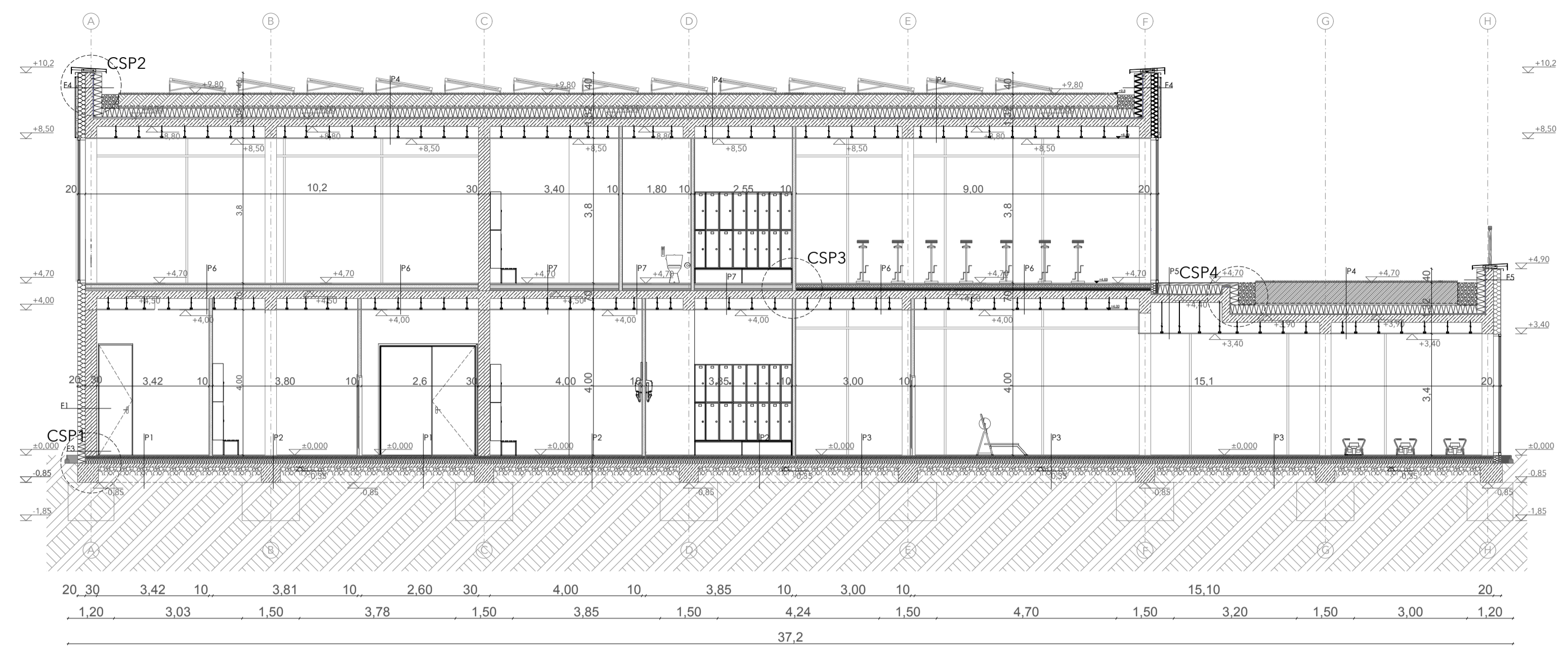
A-A metszet 1:100
